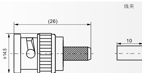
线夹
