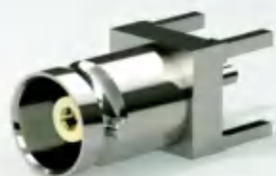
BNC-KHD1
