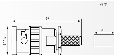
线夹
