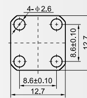
法兰盘尺寸图
