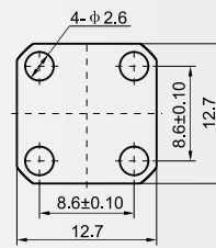
法兰盘尺寸图
