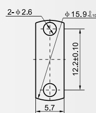
法兰盘尺寸图
