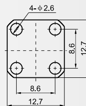
法兰盘尺寸图
