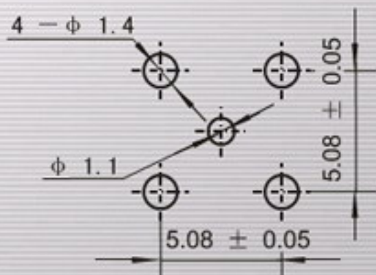
安装开孔尺寸 Mounting hole
