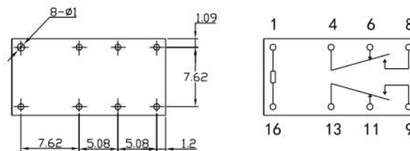
安装图
