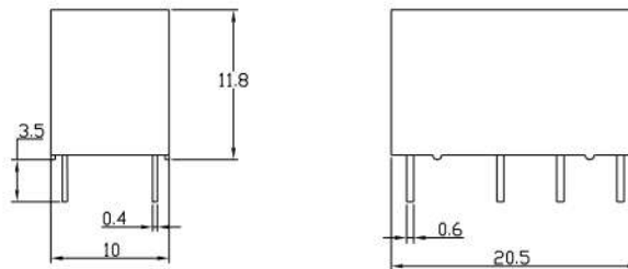
外形尺寸
