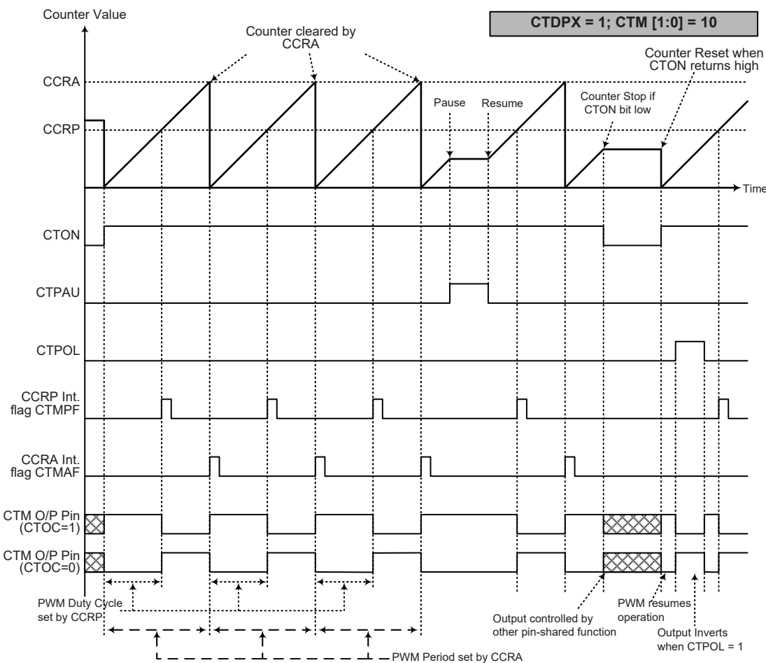
PWM Output Mode – CTD PX=1
