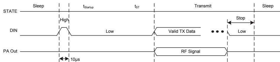
TX Enabled by DIN Input
