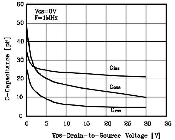
Fig. 4 C - V_{DS}
