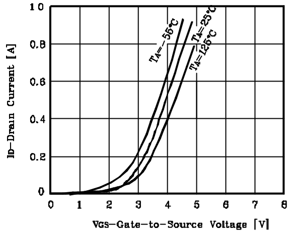
Fig. 2 I_D - V_{GS}
