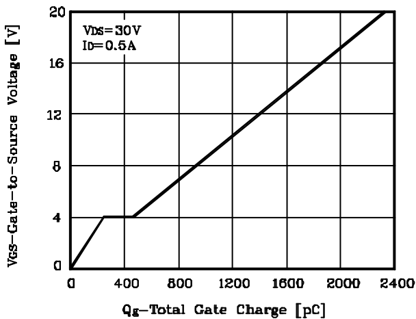
Fig. 5 V_{GS} - Q_g
