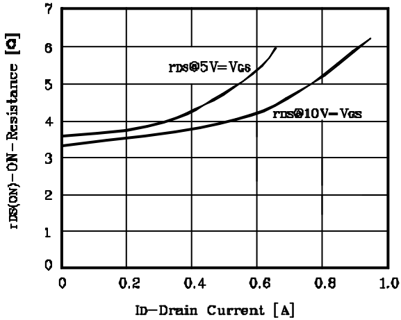
Fig. 3 R_{DS(on)} - I_D
