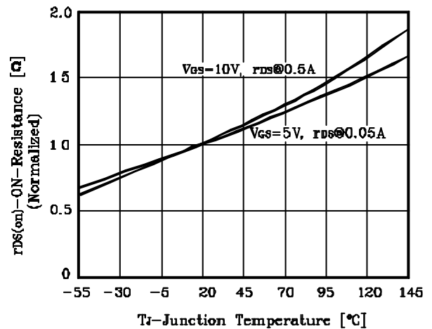
Fig. 6 R_{DS(on)} - T_J
