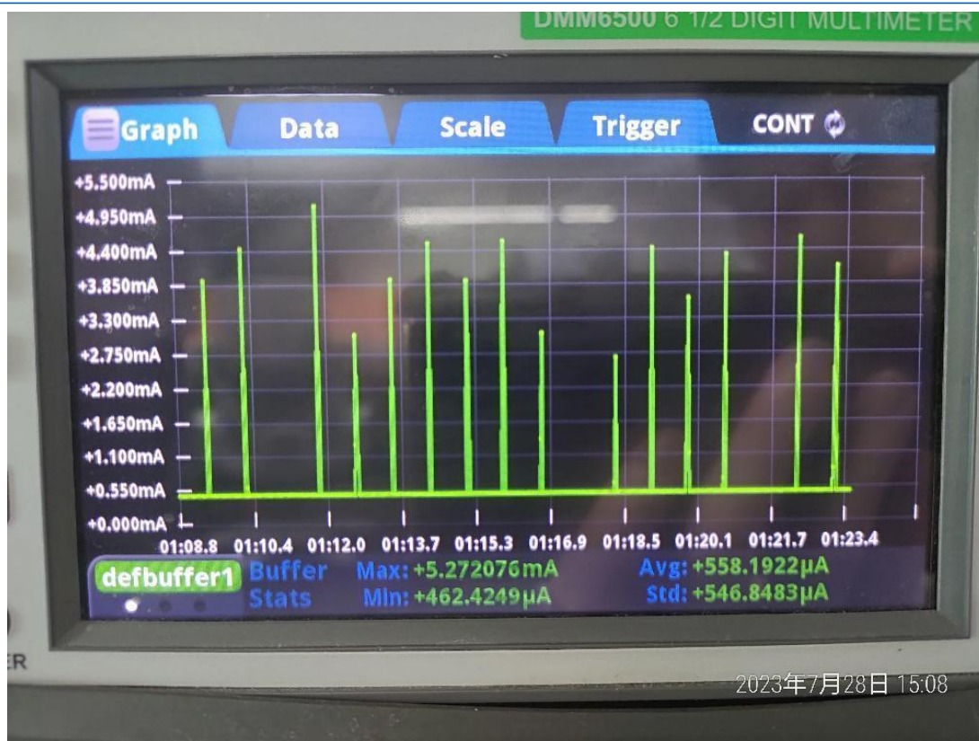
图 8 使能低功耗休眠状态下的工作电流图示
