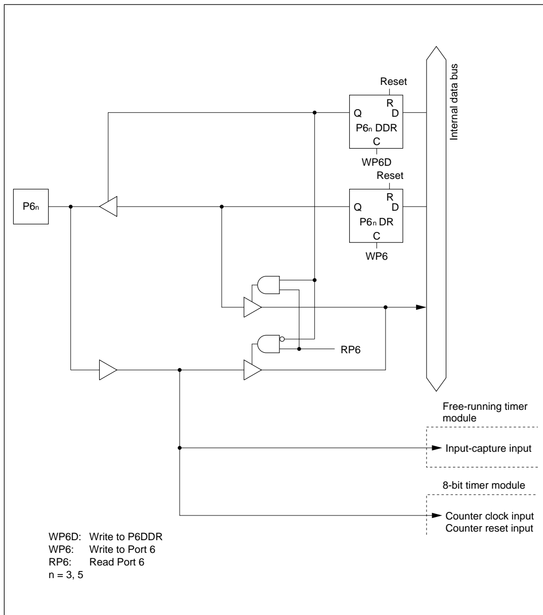
Figure C-6 (d) Port 6 Block Diagram (Pins P6 3 and P6 5 )
