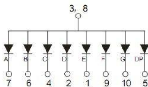
数码管显示及引脚位置图
