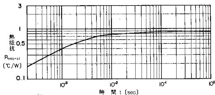
過渡熱抵抗(ダイオード)特性
