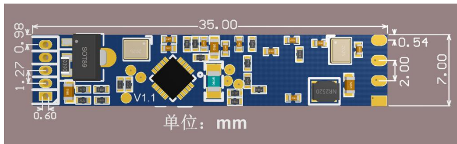
图 5 模块尺寸图
