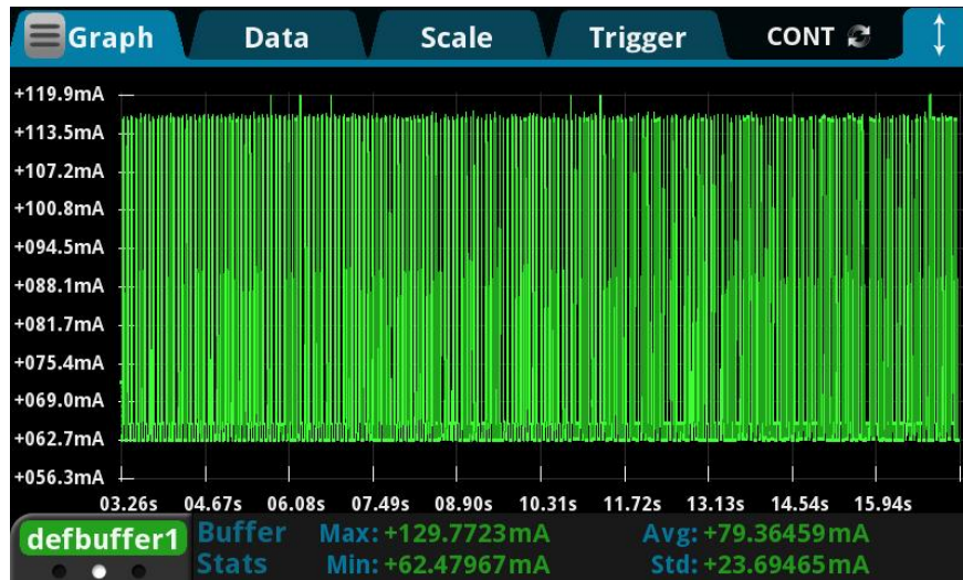
图 11 模块工作电流实测数据
