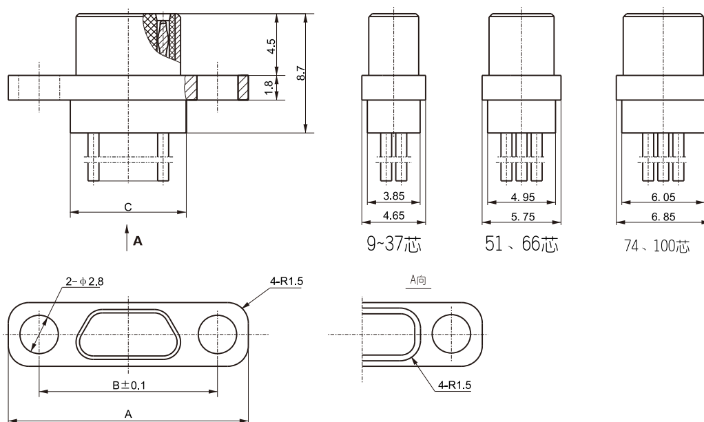
产品外形尺寸图
