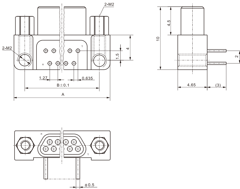
产品外形尺寸图
