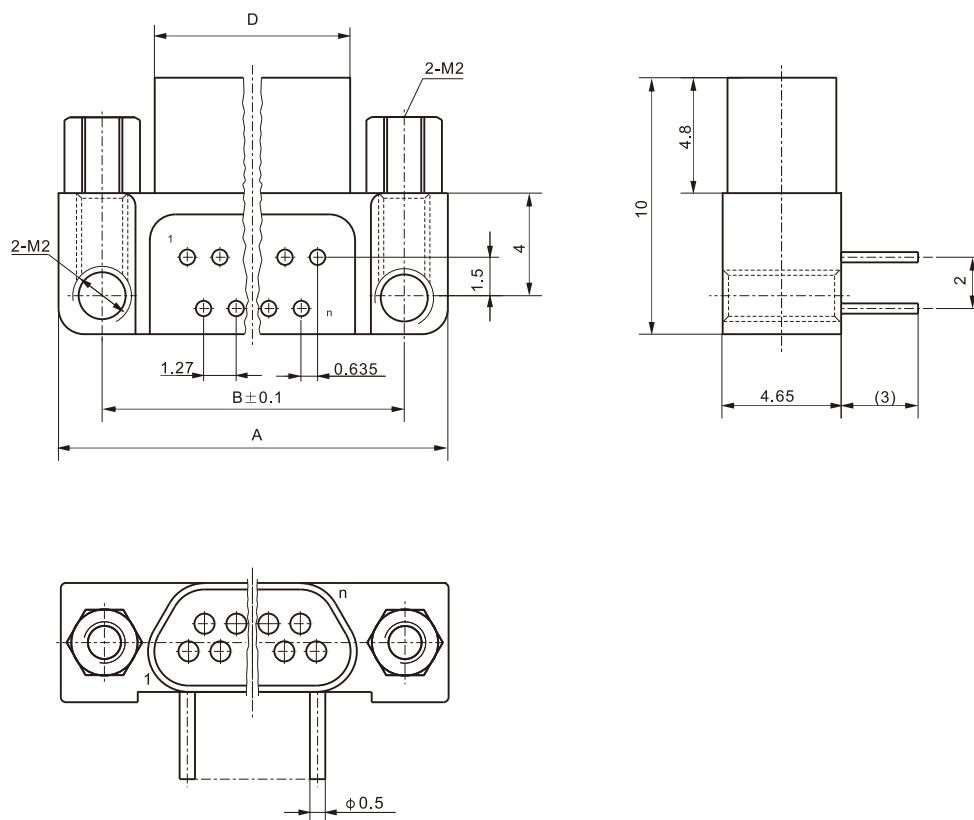
产品外形尺寸图
