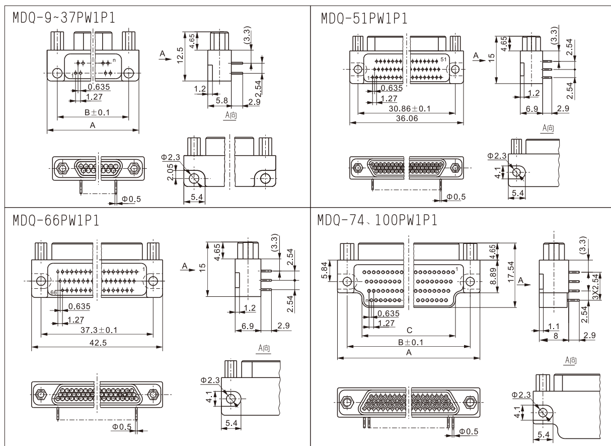
产品外形尺寸图
