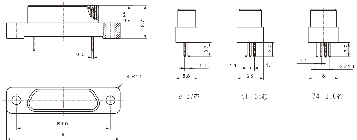
产品外形尺寸图
