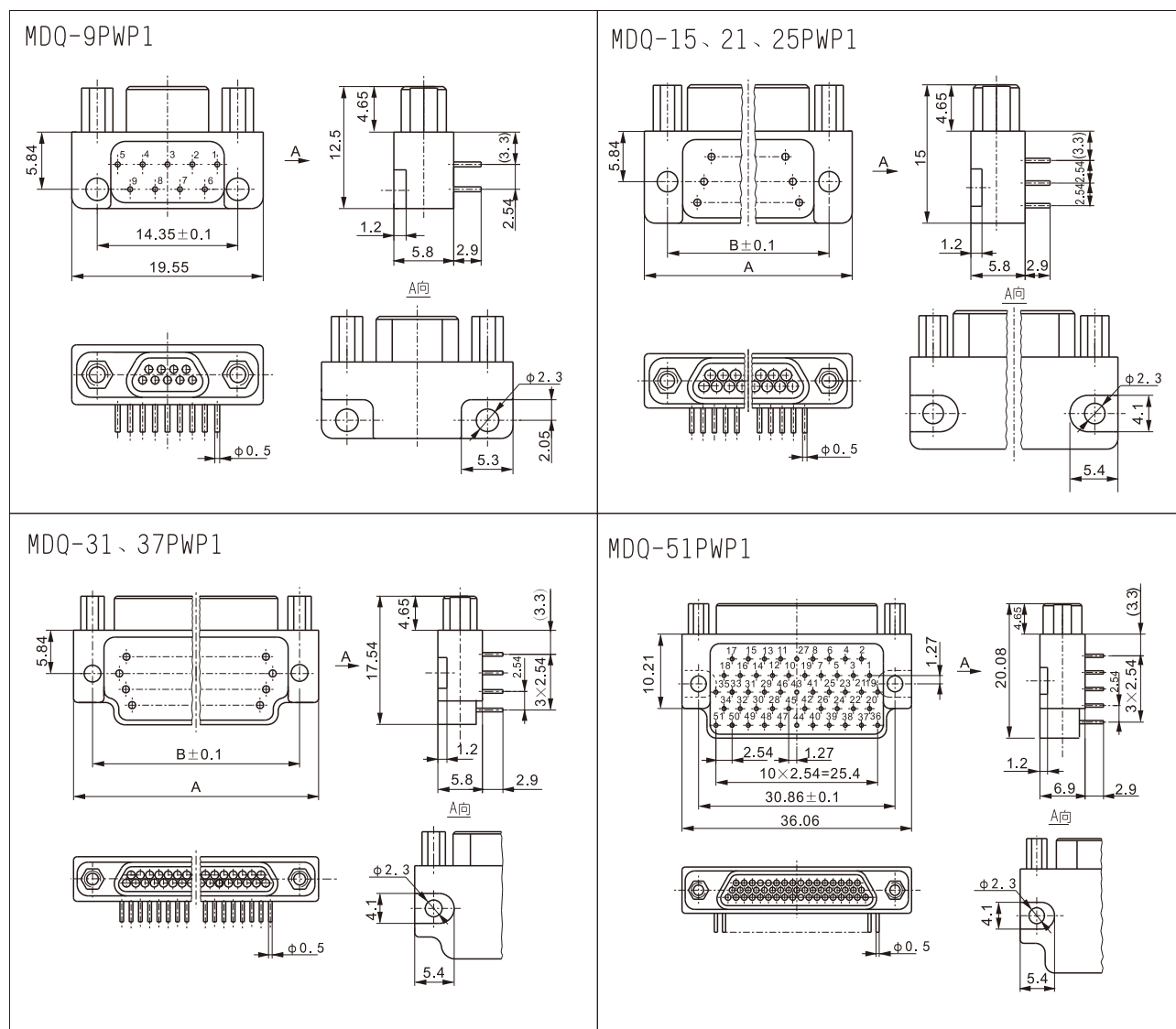
产品外形尺寸图
