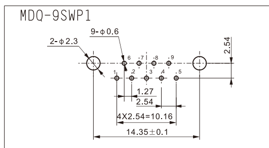
MDQ弯式焊印制板式W型插孔电连接器开孔尺寸
