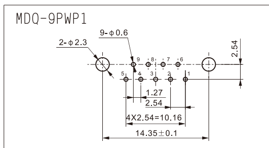
MDQ弯式焊印制板式W型插针电连接器开孔尺寸
