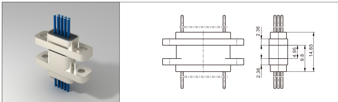
产品对接后尺寸图
