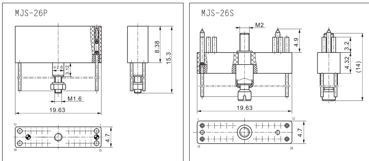
产品外形尺寸图
