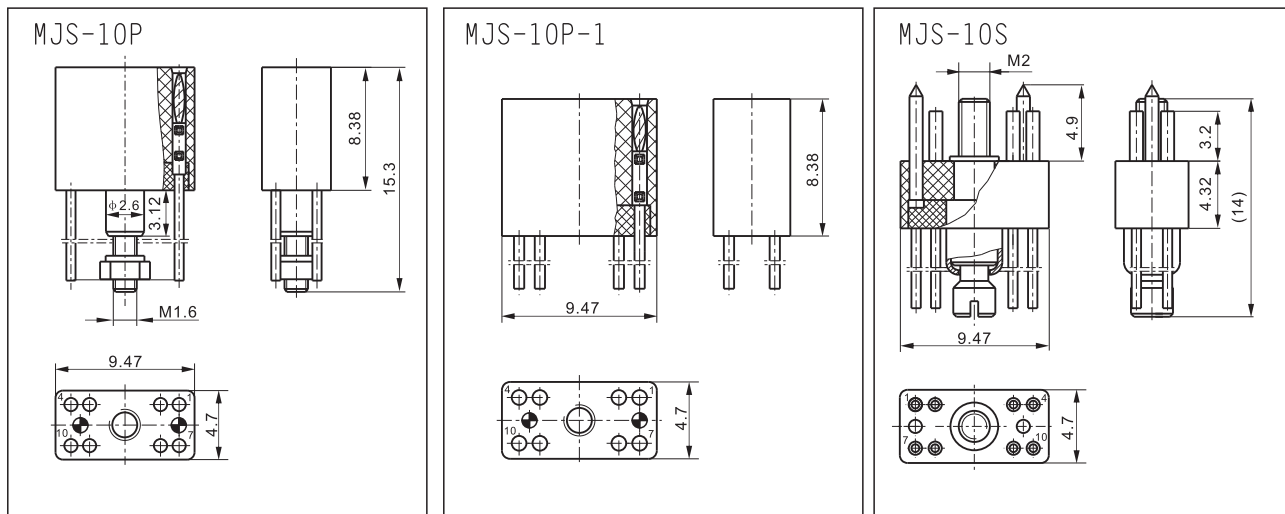
产品立体图
