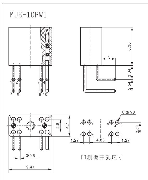
产品外形尺寸图
