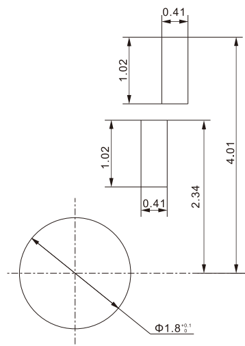
引脚封装尺寸局部放大图
