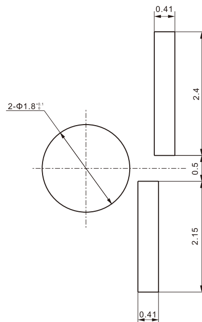
引脚封装尺寸局部放大图
