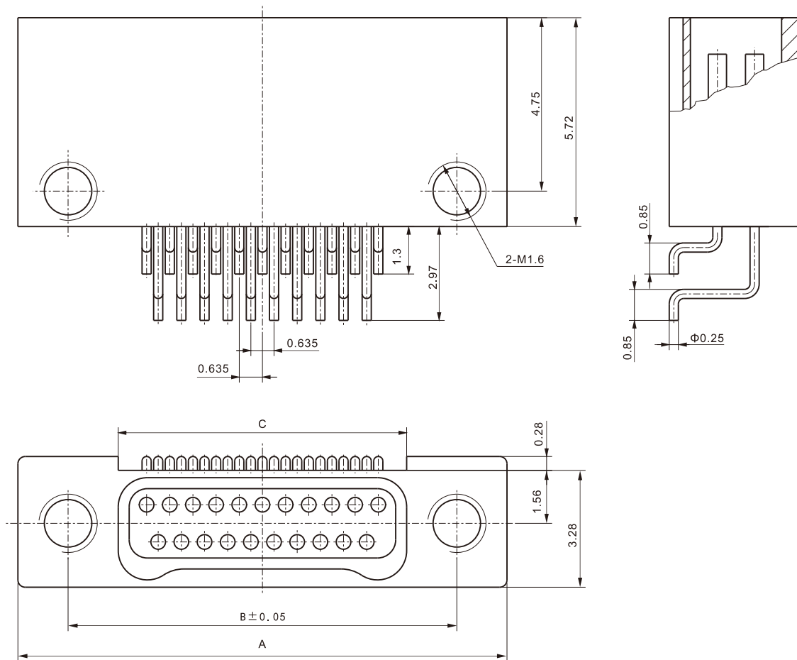
产品尺寸图
