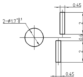
引脚封装尺寸局部放大图
