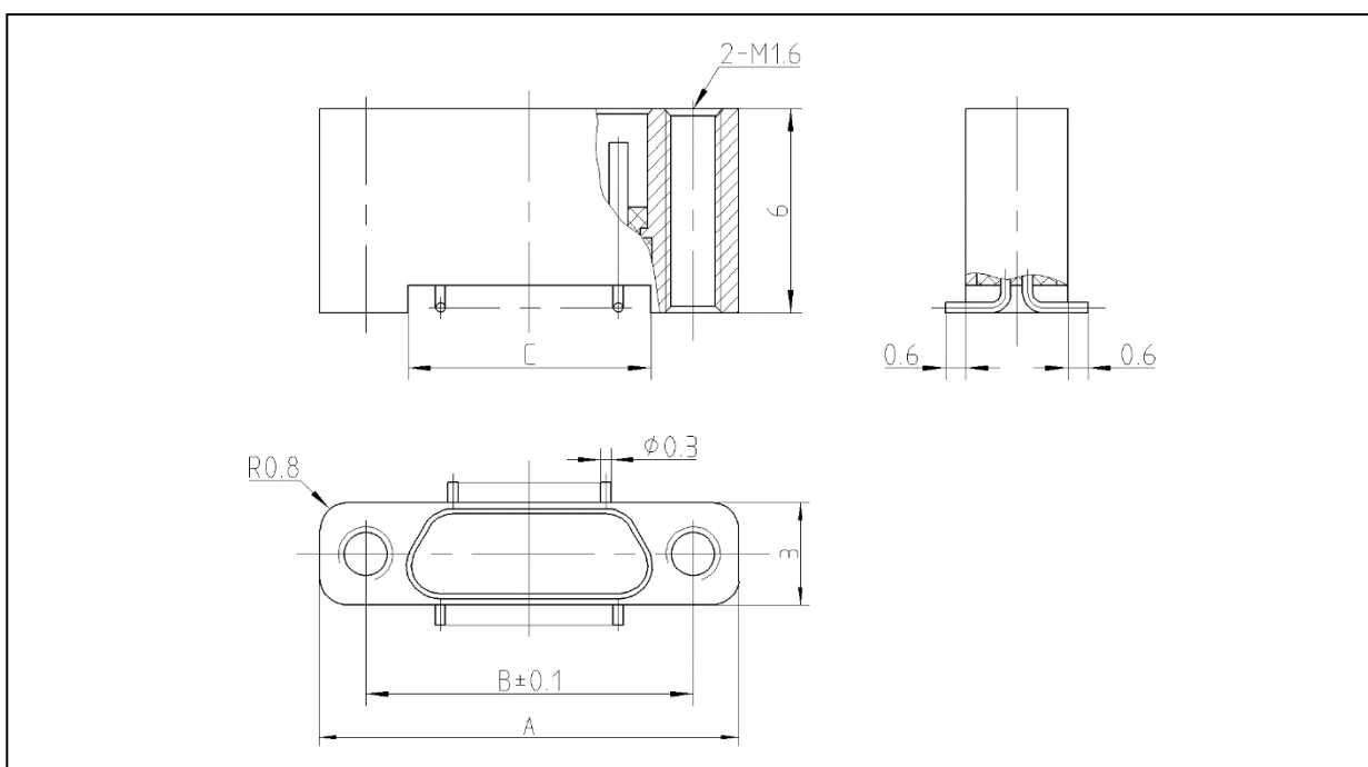
产品外形尺寸图
