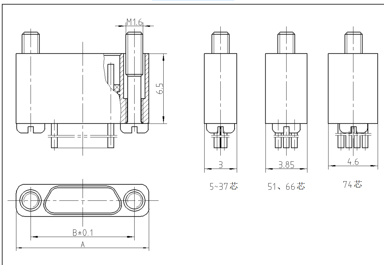
产品外形尺寸图
