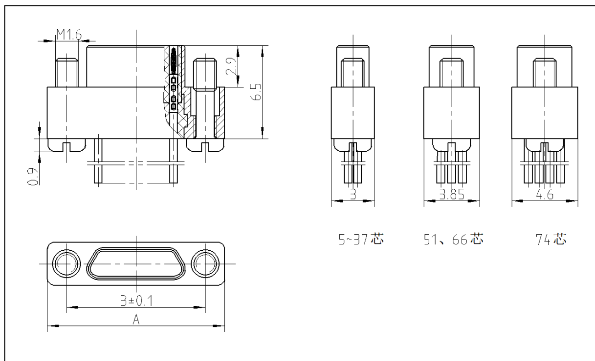
产品外形尺寸图
