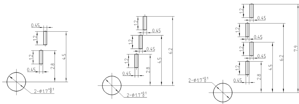
引脚封装尺寸局部放大图
