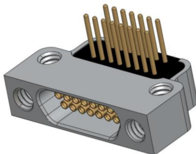
产品外形尺寸图
