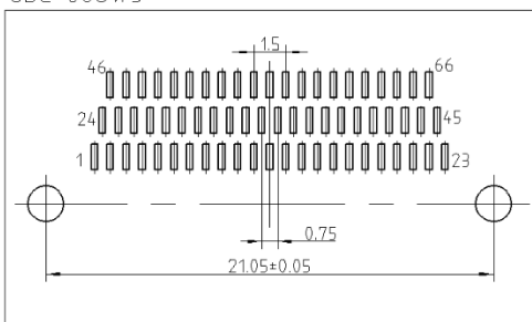
引脚封装尺寸局部放大图
