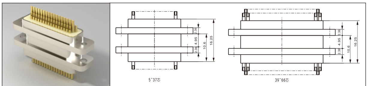
产品对插后尺寸图
