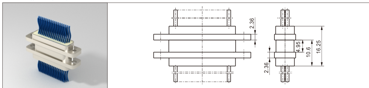
产品对插后外形图
