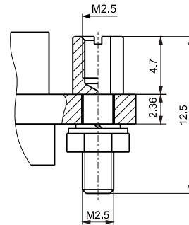
外形尺寸
