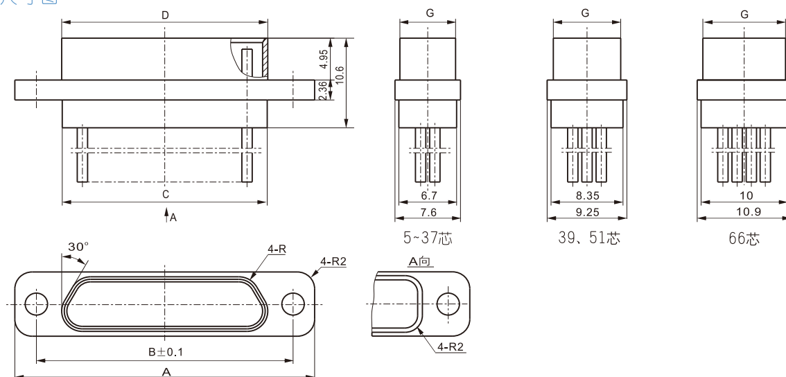
产品外形尺寸图
