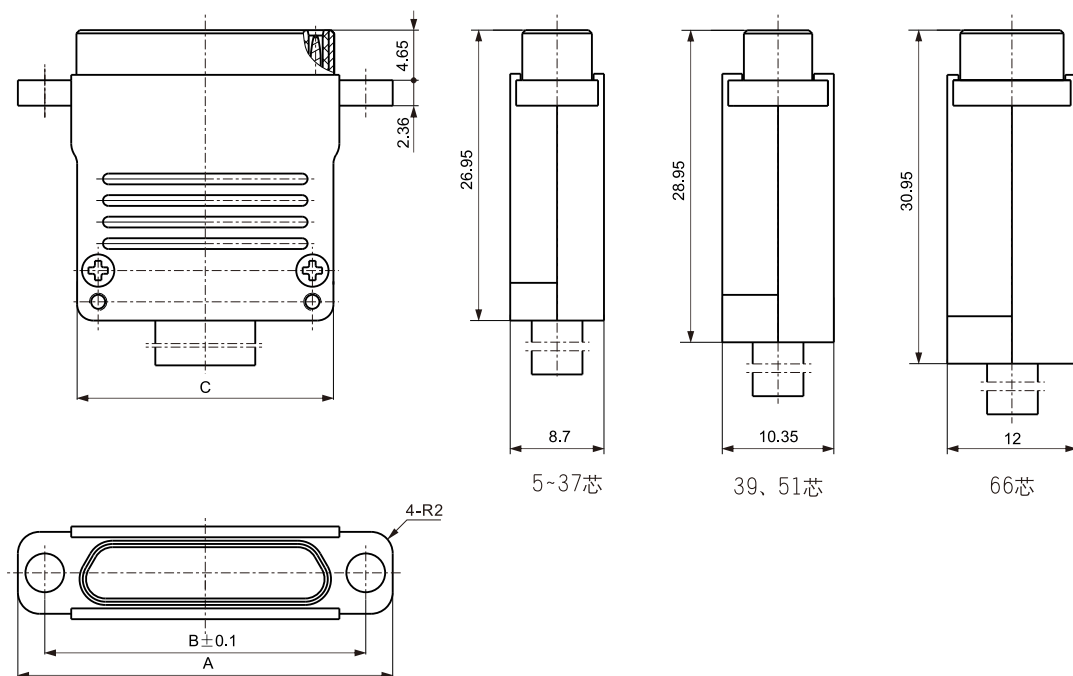
产品外形尺寸图
