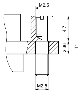
外形尺寸
