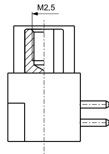
外形尺寸
