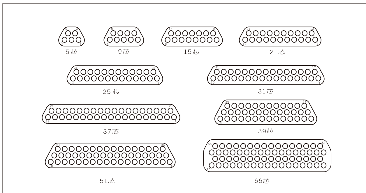
型谱排列(从插针连接器对插面看)
