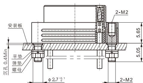
ZMDC-PP 产品安装 P 型附件参考示例
