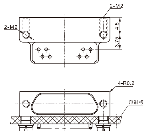
ZMDC-SW 弯式焊印制板式插孔连接器安装参考示例
