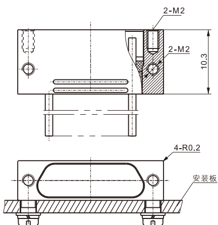
ZMDC-S1 产品水平安装参考示例
