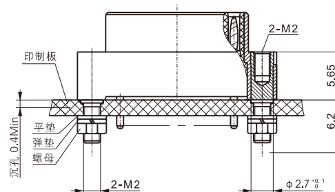
ZMDC-PNP 产品安装 P 型附件参考示例
