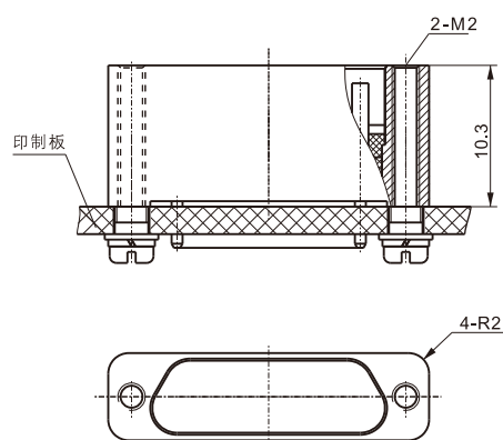
ZMDC-SN/SN1 产品垂直安装参考示例
