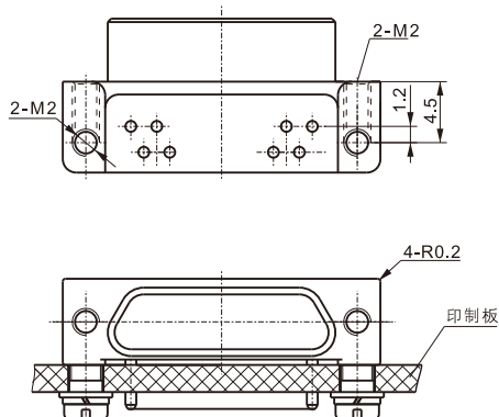
ZMDC-PW 弯式焊印制板式插针连接器安装参考示例
