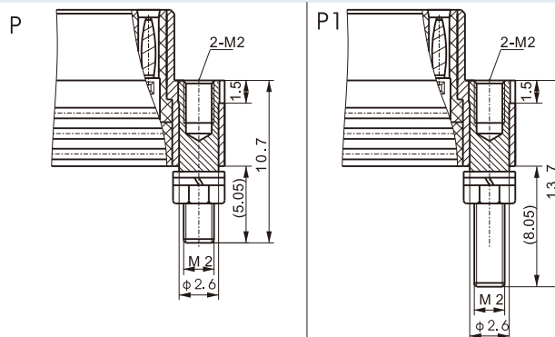
外型尺寸
