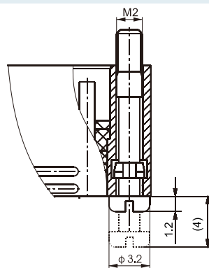
L5型附件尺寸
