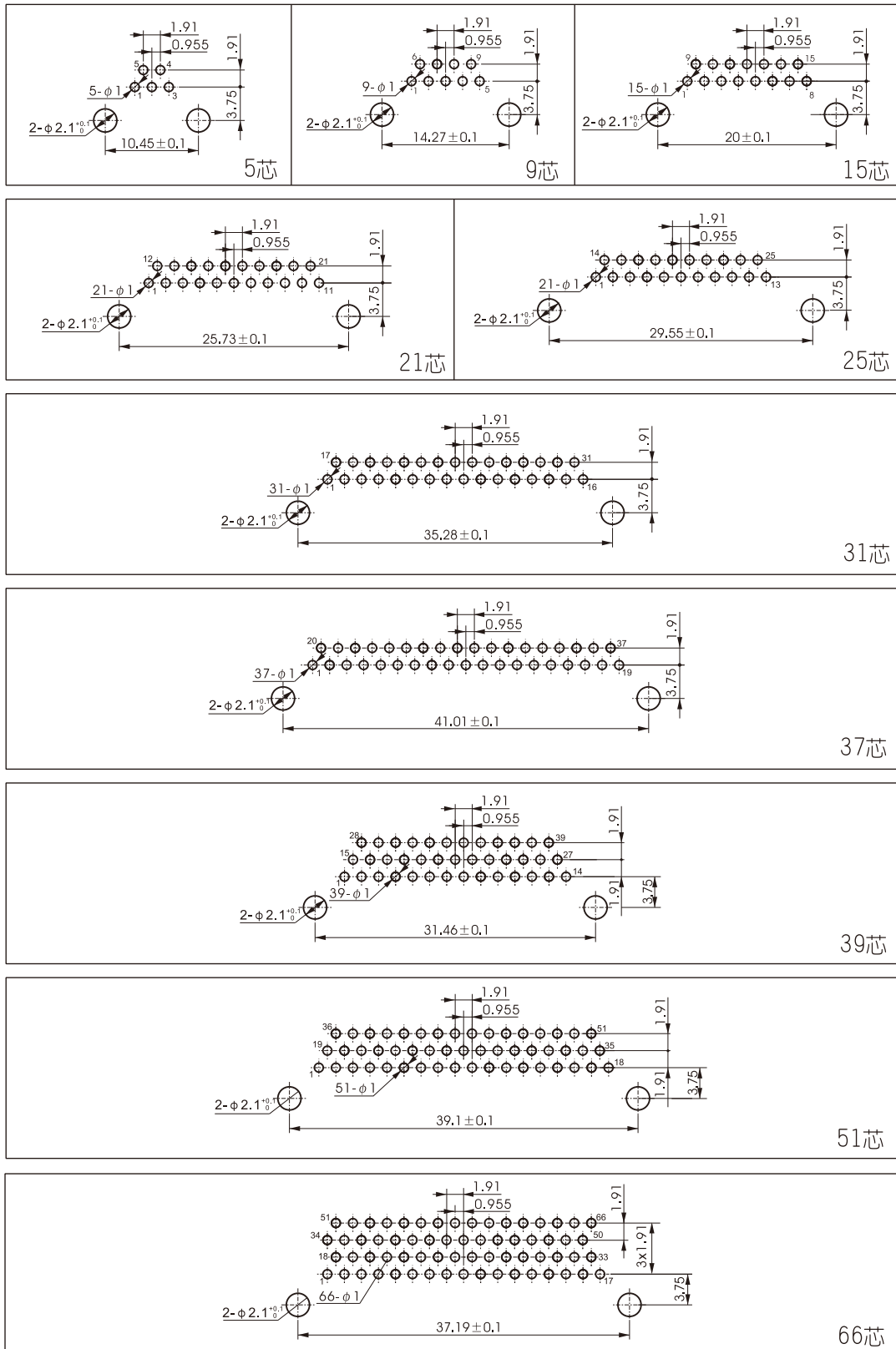
弯式焊印制板式插孔电连接器印制板开孔尺寸
