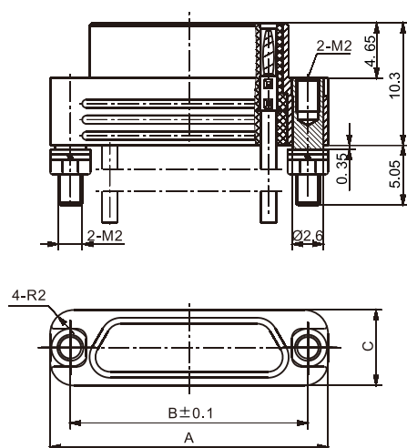
产品外形尺寸图
