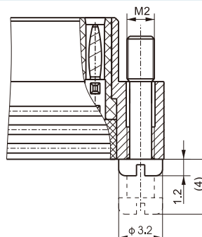
L型附件尺寸
