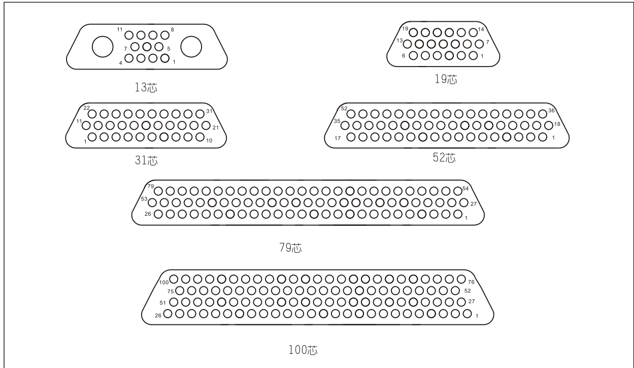
型谱排列(从插座对插面看)
