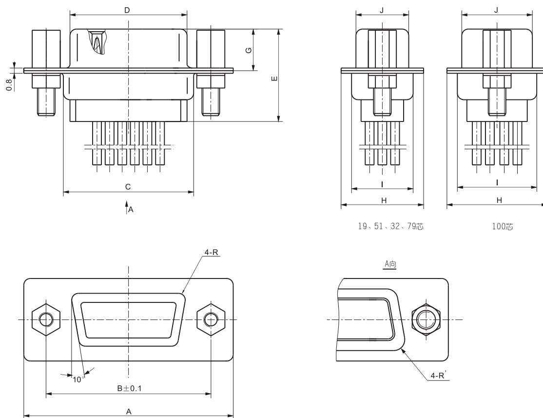
产品外形尺寸图
