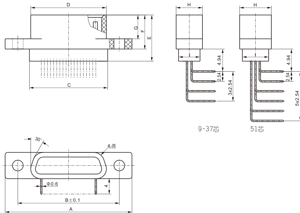
产品外形尺寸图
