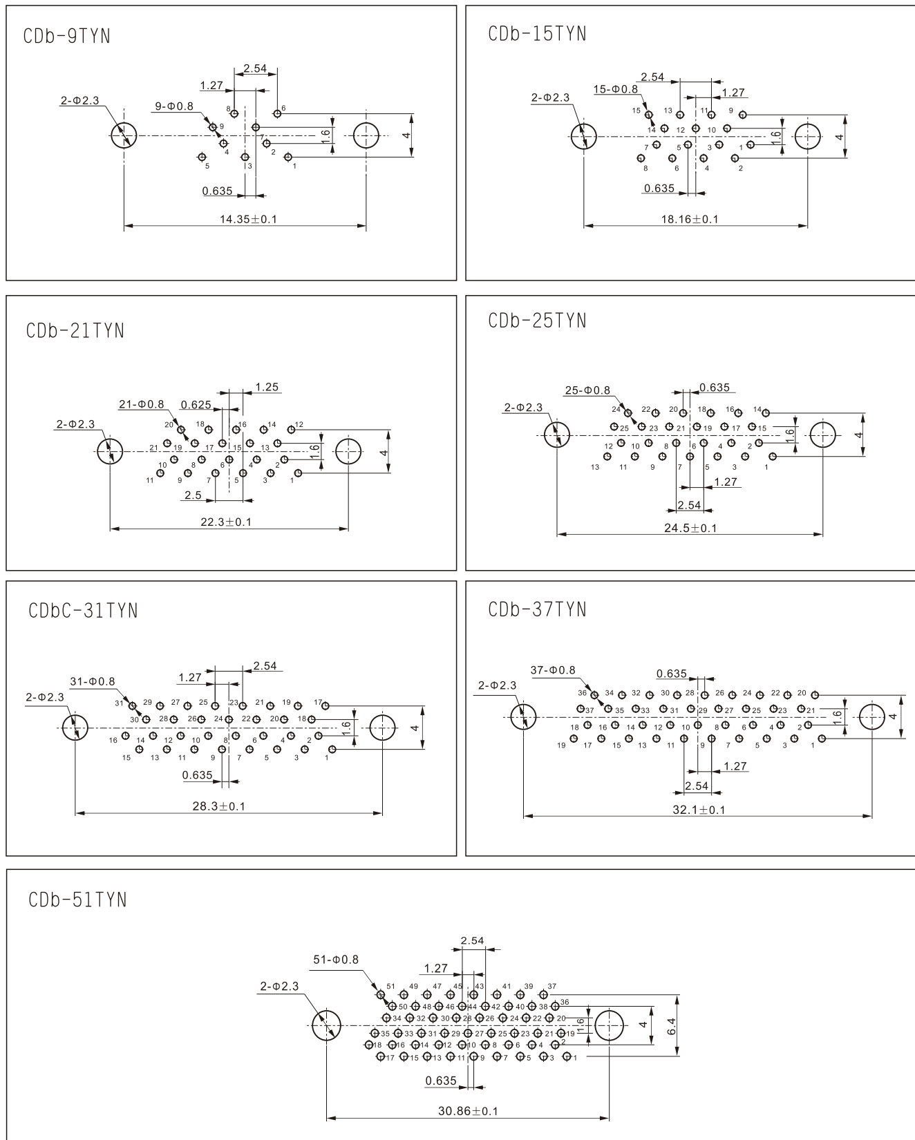
Cdb直式焊印制板式N型插针电连接器开孔尺寸
