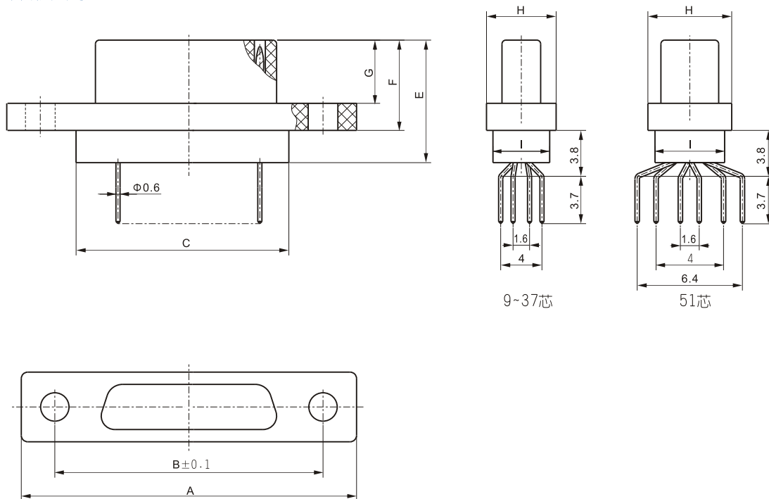
产品外形尺寸图
