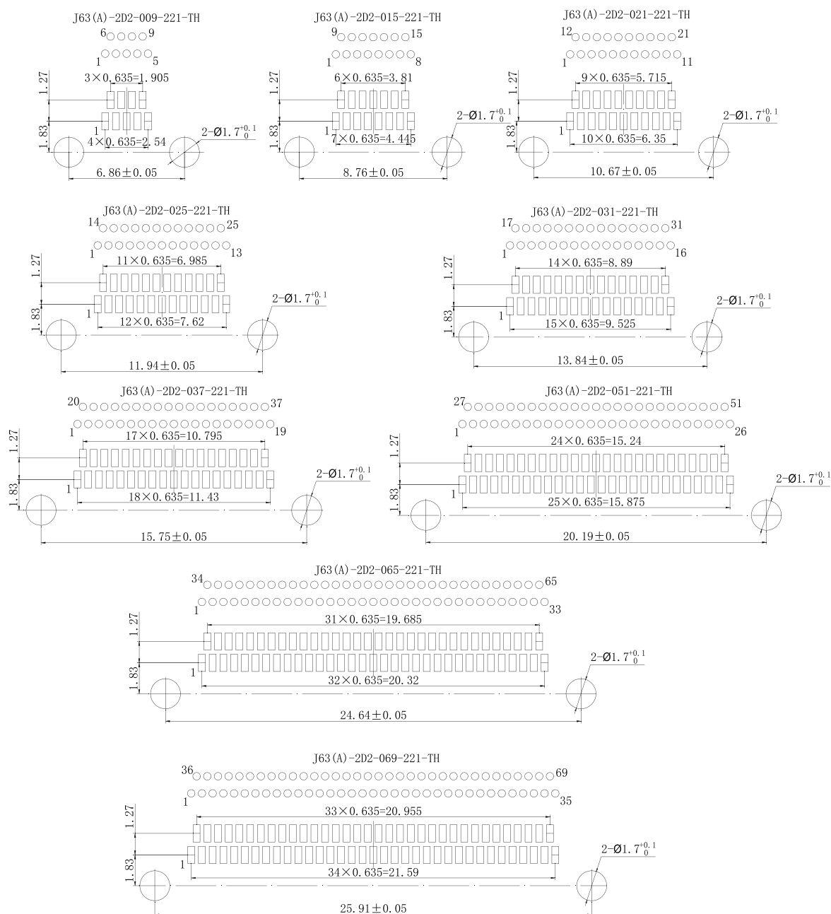
封装尺寸局部放大图
