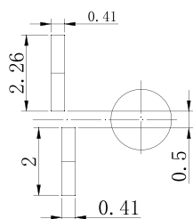
引脚封装尺寸局部放大图
