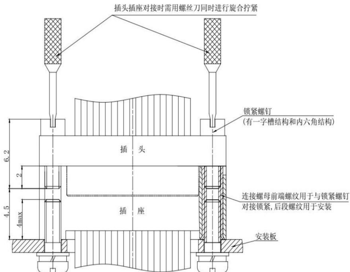
插头、插座连接锁紧、安装示意图
