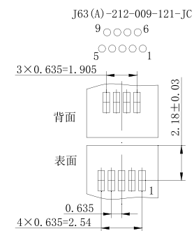
封装尺寸局部放大图
