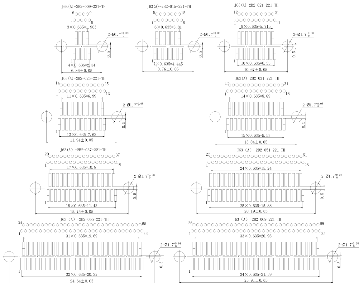
引脚封装尺寸局部放大图
