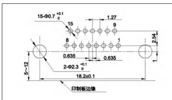
J30J-15TJW-J
