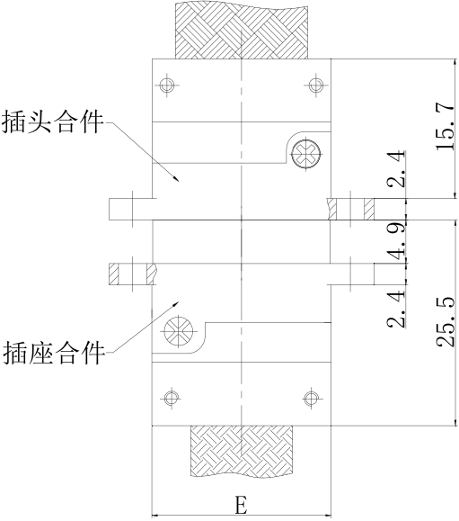
J30J-74~100 芯
