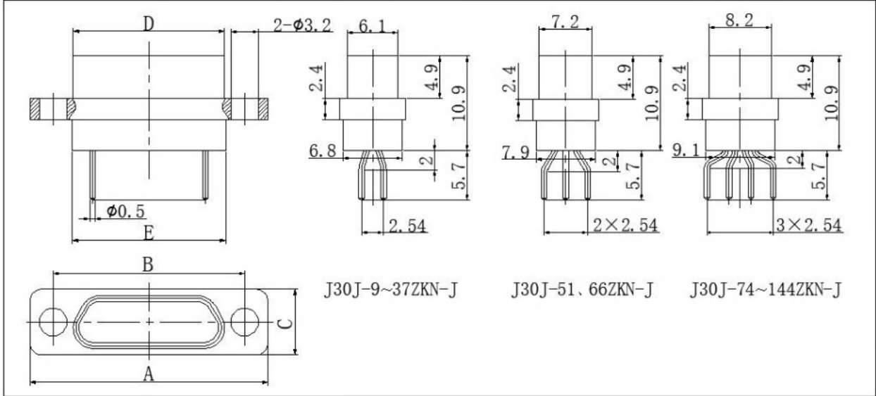
J30J 插装印制板基本型\直插印制板 N-J 型\ J30J-TJN-J&J30J-ZKN-J
