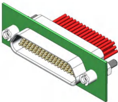
组装示意图
