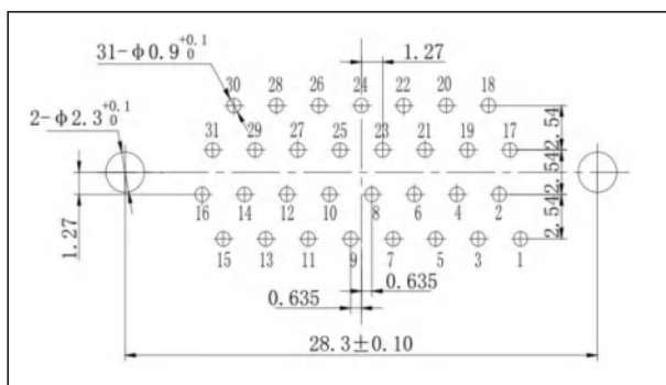
J30J-31TJN□
