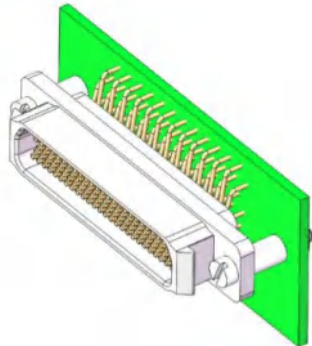
组装示意图
