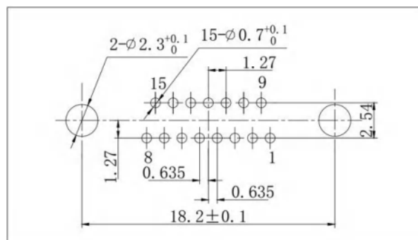
J30JR-15ZJN-J
