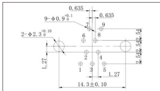
J30J-9ZKN□
