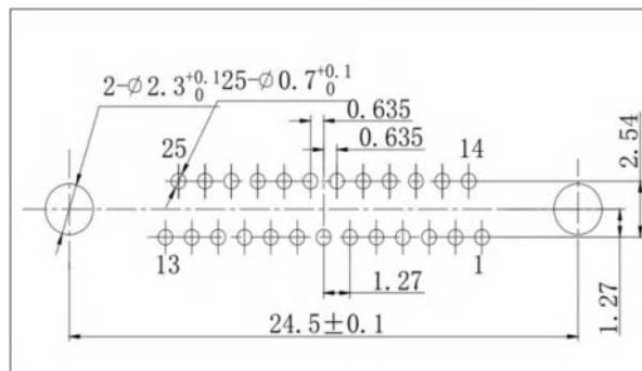
J30JR-25ZJN-J
