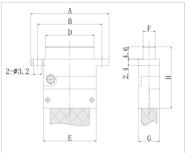
J30J-□TJ-A
