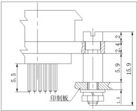
产品外形尺寸图
