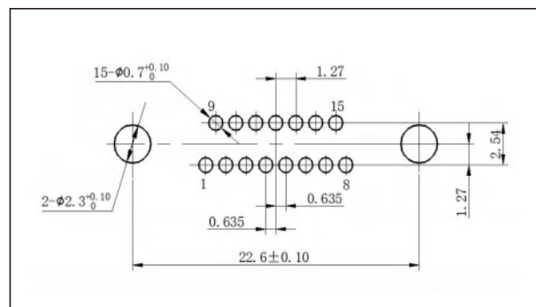
J30JA-15ZKN-J
