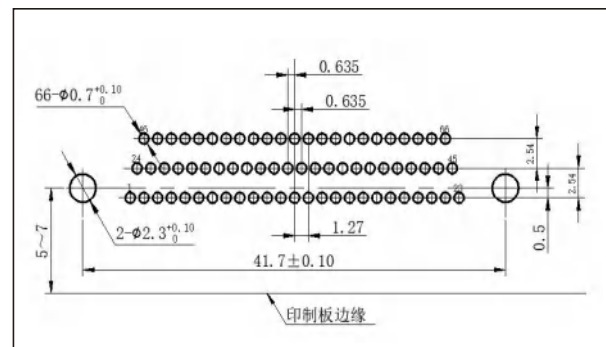
J30JA-66ZKW-J
