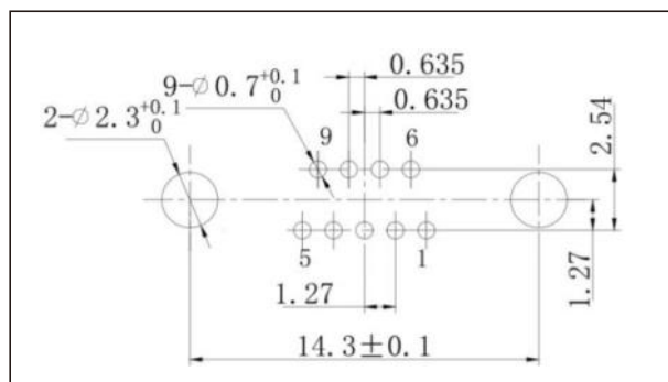
J30J-9TJN□-J
