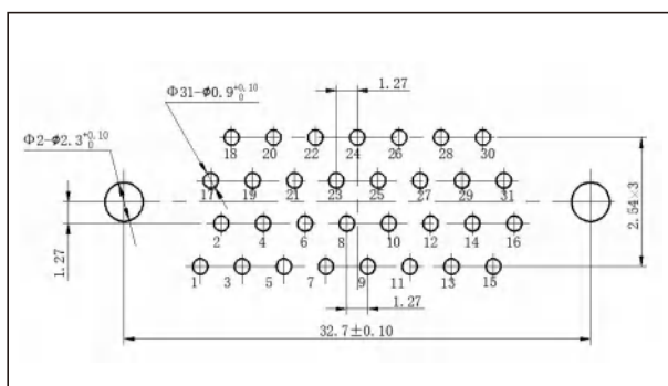
J30JA-31ZKN
