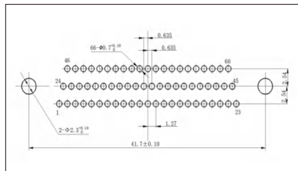
J30JA-66ZKN-J
