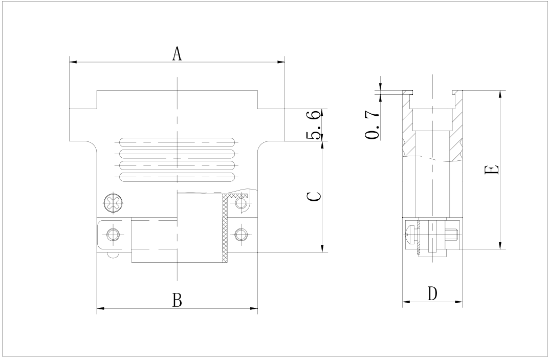
A3 型线夹合件的尺寸
