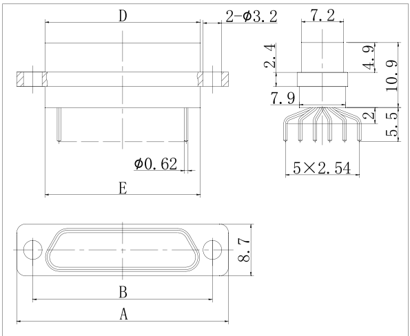
J30J-51、66ZKN
