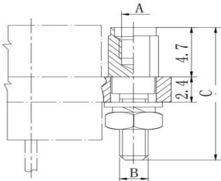
产品外形尺寸图
