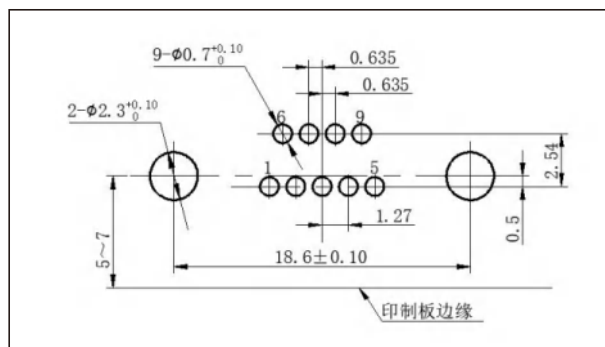
J30JA-9ZKW-J
