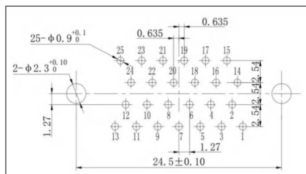
J30J-25TJN□
