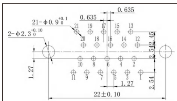
J30J-21TJN□
