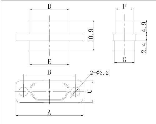
J30JR-□ZJ
