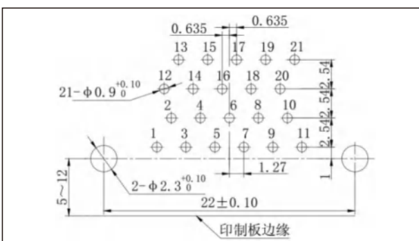
J30J-21ZKW
