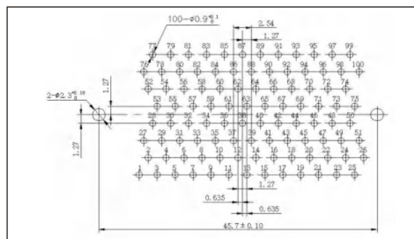
J30J-100ZKN□
