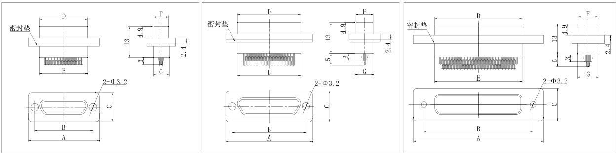
J30JM-9~37ZKS
