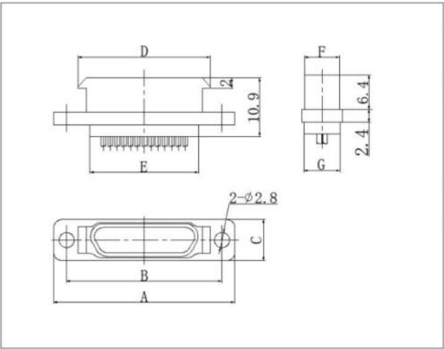
J30JA-□ZK
