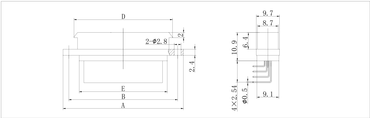
J30JA-74、100ZKW-J
