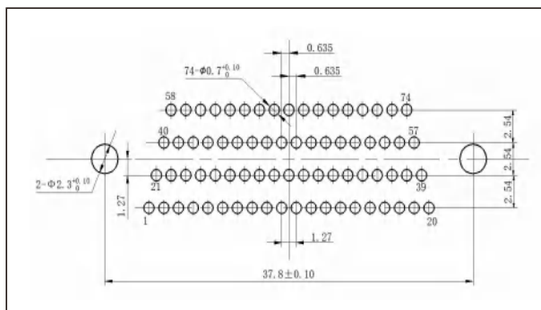
J30JA-74ZKN-J
