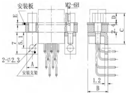
产品外形尺寸图
