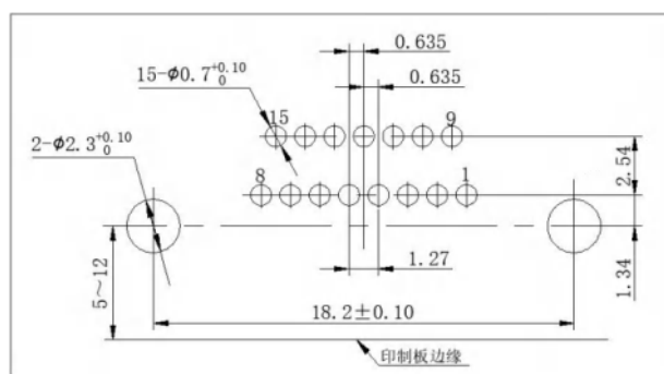
J30JR-15ZJW-J
