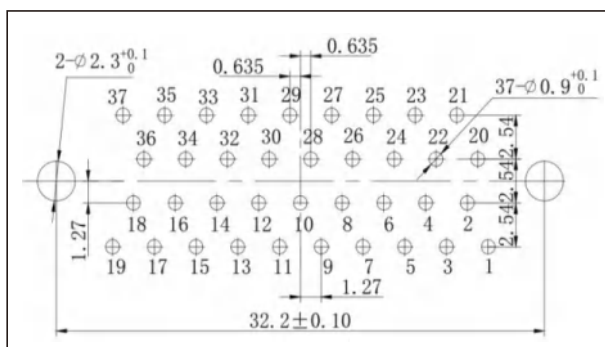
J30J-37TJN□
