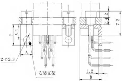
产品外形尺寸图
