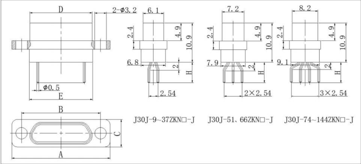
产品外形尺寸和各芯数插座的左视图
