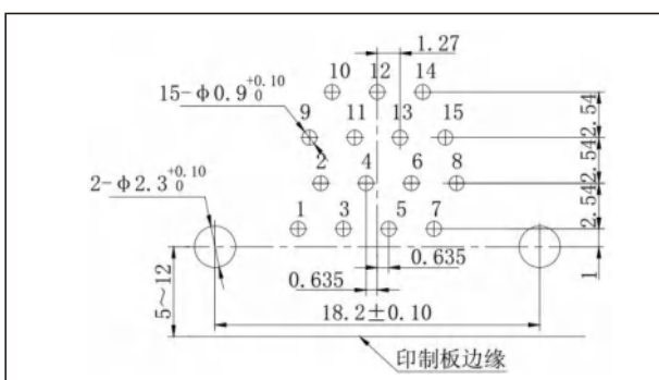
J30J-15ZKW
