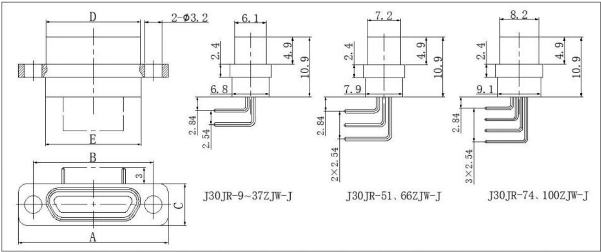
产品外形尺寸和各芯数插座的左视图
