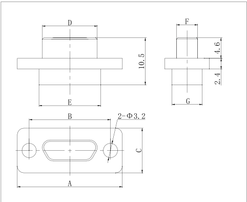
J30J-□TJ-Q8
