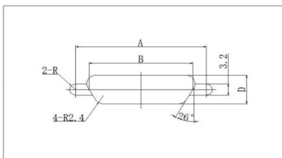
板后安装开孔尺寸 (100 芯除外)
