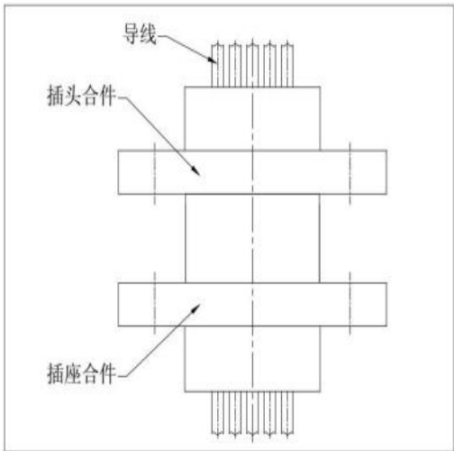
主视图
