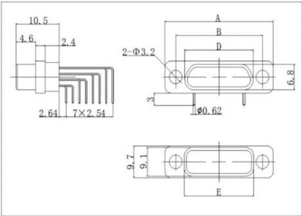
J30J-74~144TJW
