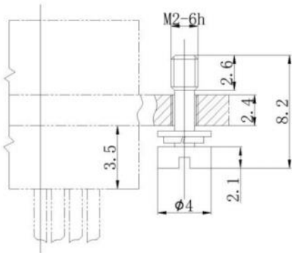
产品外形尺寸图
