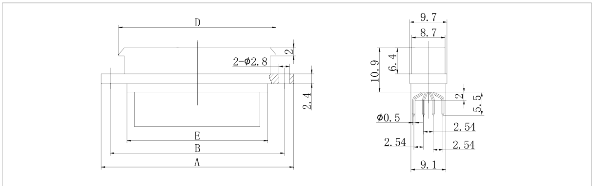
J30JA-74、100ZKN-J
