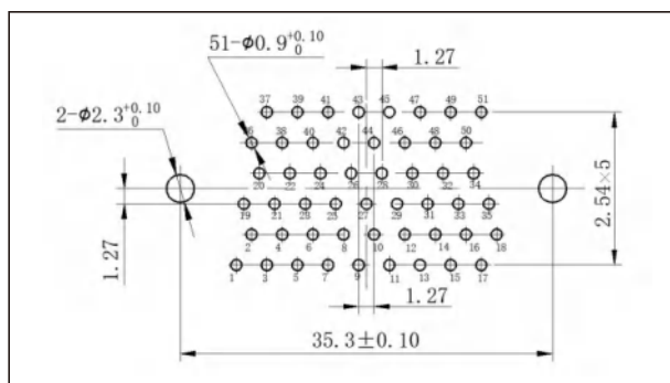
J30JA-51ZKN
