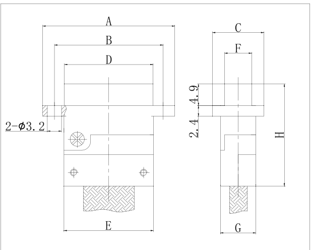
产品外形尺寸图
