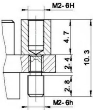
产品外形尺寸图
