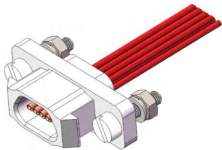
组装示意图
