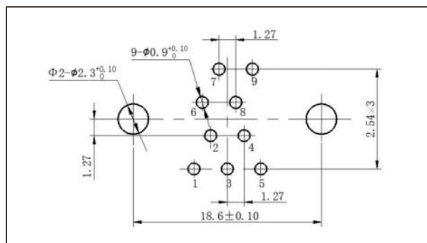
J30JA-9ZKN
