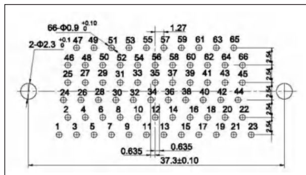
J30J-66ZKN□
