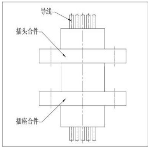
主视图
