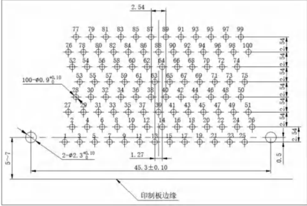
J30JA-100ZKW
