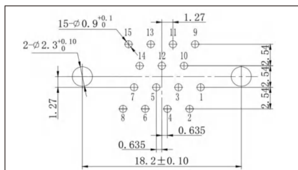
J30J-15TJN□
