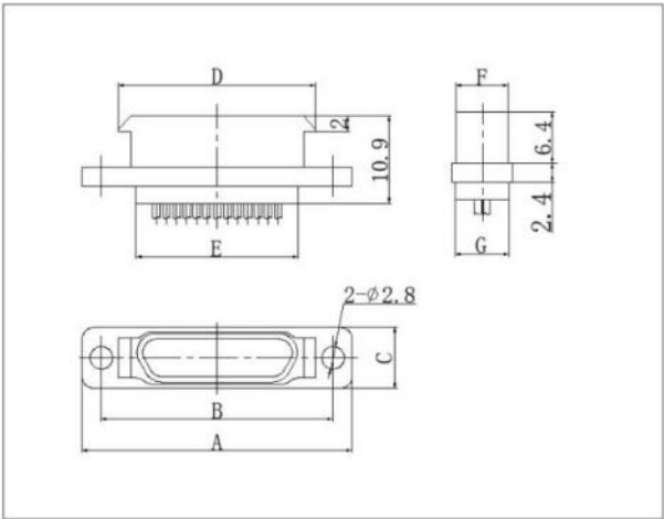
产品外形尺寸图
