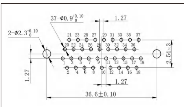
J30JA-37ZKN
