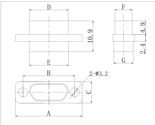
J30J-□ZK
