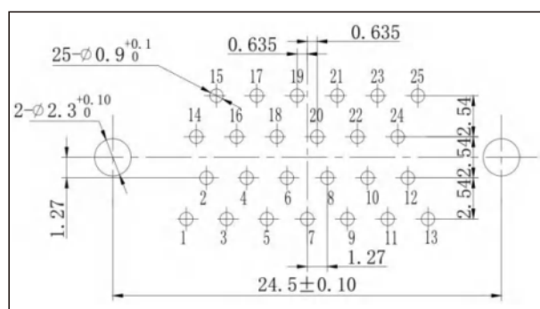
J30J-25ZKN□
