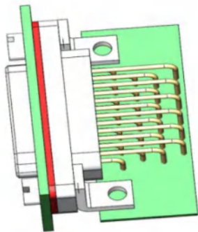
组装示意图
