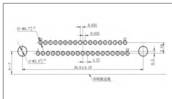
J30JA-37ZKW-J
