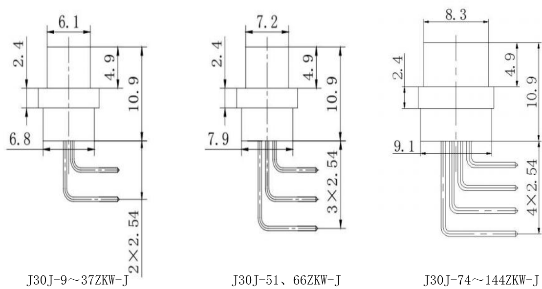
J30J-9~1144ZKW-J 各芯数插座合件的左视图
