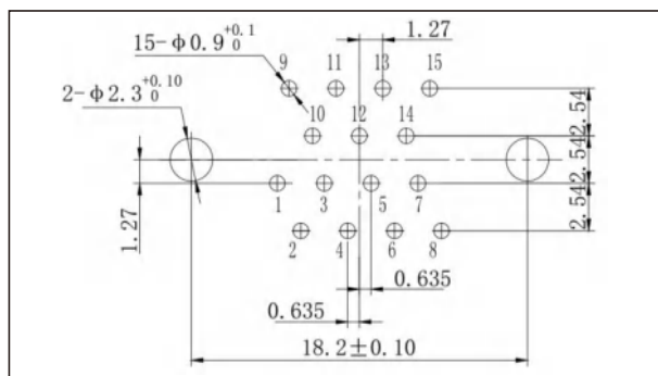
J30J-15ZKN□
