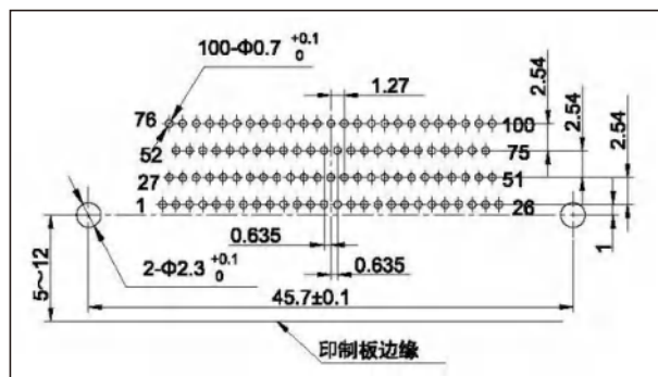
J30J-100ZKW-J
