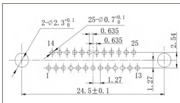
J30J-25ZKN□-J
