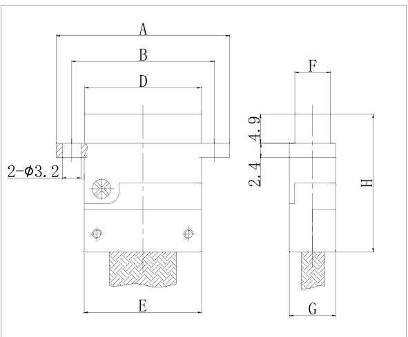
J30J-□ZK-A
