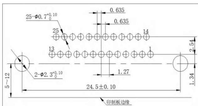
J30JR-25ZJW-J
