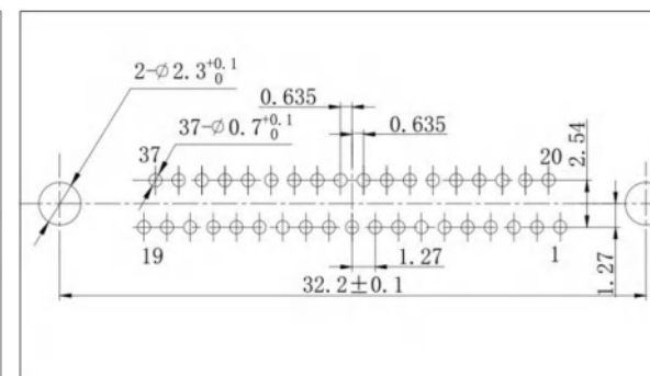
J30JR-37ZJN-J
