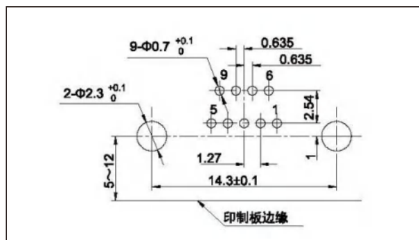
J30J-9TJW-J
