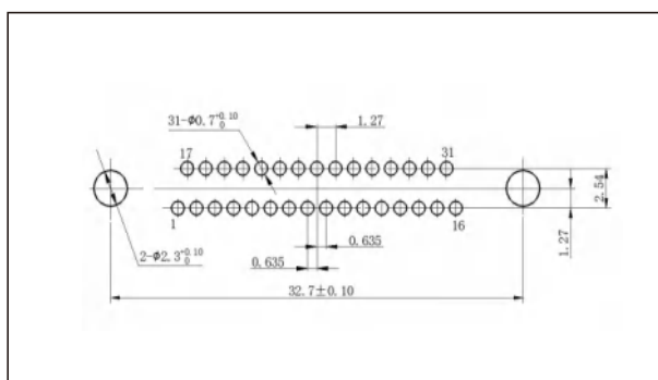
J30JA-31ZKN-J
