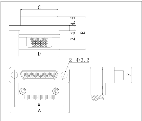
J30J-□TJ-C1
