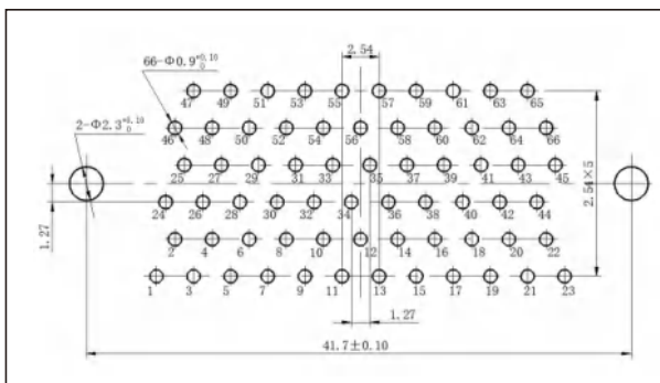
J30JA-66ZKN
