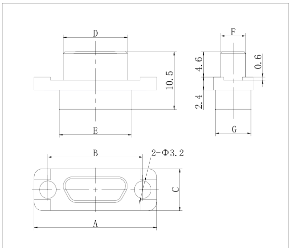
J30J-□TJ-D
