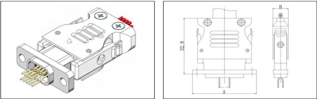
产品对接后外形尺寸
