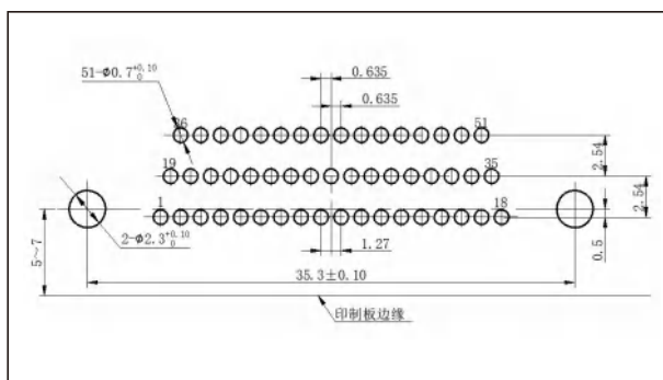
J30JA-51ZKW-J
