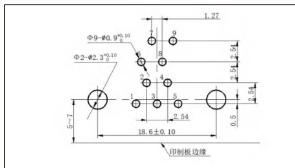
J30JA-9ZKW
