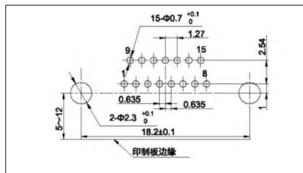
J30J-15ZKW-J
