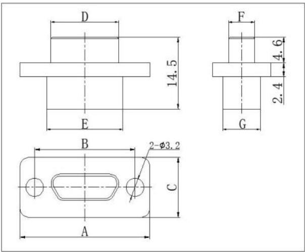
J30JM-□TJ
