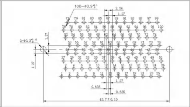
J30JA-100ZKN
