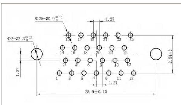
J30JA-25ZKN
