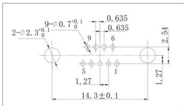
J30JR-9ZJN-J
