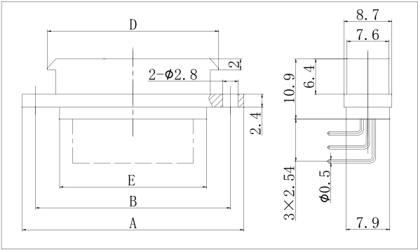
J30JA-51、66ZKW-J
