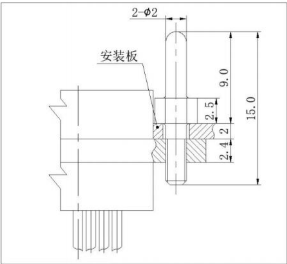
产品外形尺寸图
