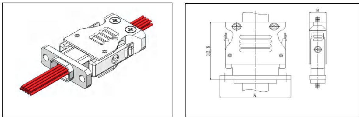
产品对接后外形尺寸
