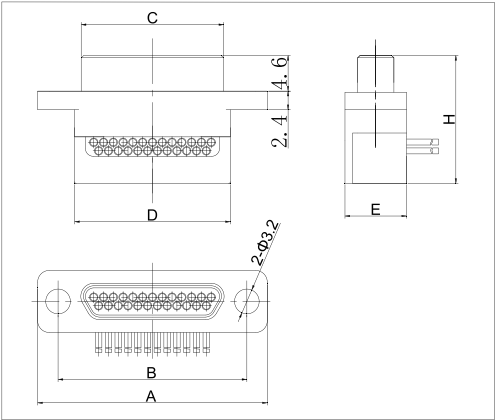
J30J-□TJ-C
