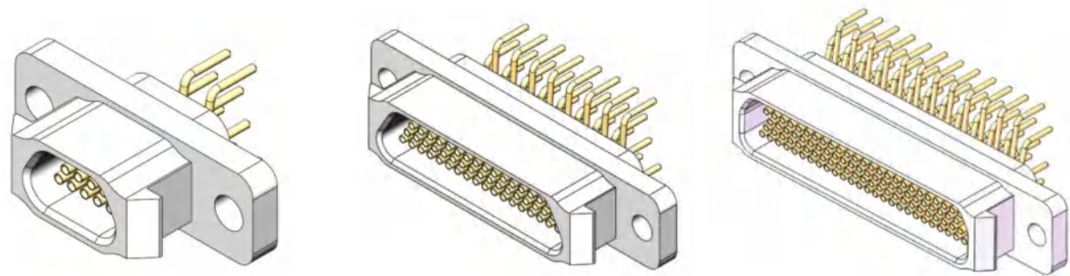
J30JA-9ZKN
