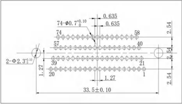
J30JR-74ZJN-J
