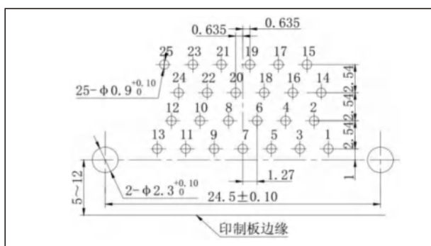
J30J-25TJW
