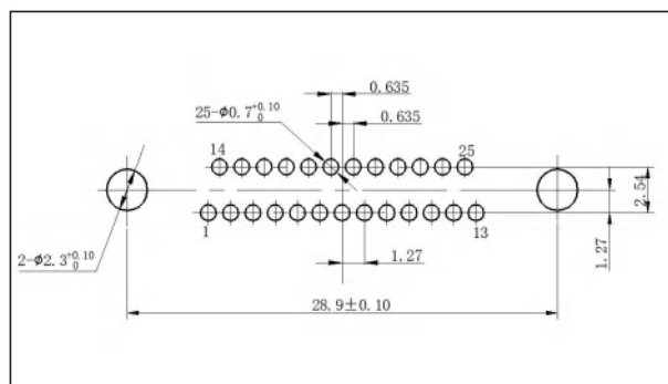
J30JA-25ZKN-J
