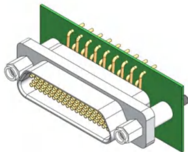
组装示意图
