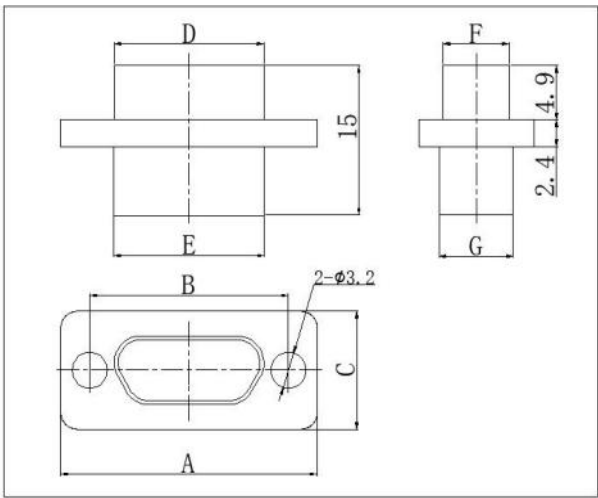
J30JM-□ZK
