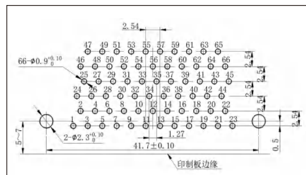
J30JA-66ZKW
