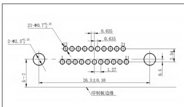
J30JA-21ZKW-J
