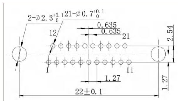
J30J-21ZKN□-J
