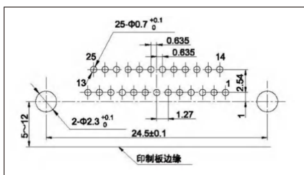
J30J-25TJW-J
