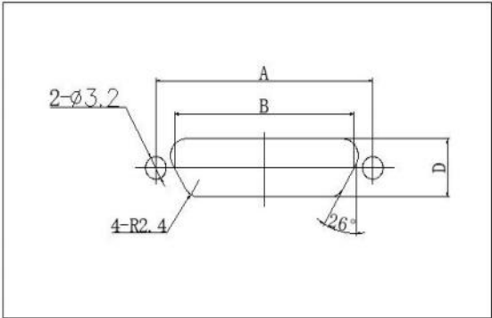
板后安装开孔尺寸
