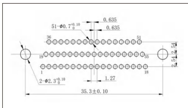
J30JA-51ZKN-J
