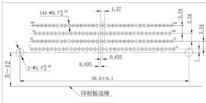
J30J-144ZKW-J
