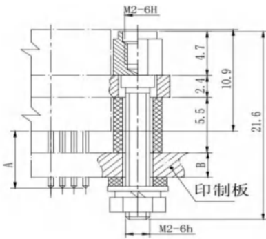
产品外形尺寸图
