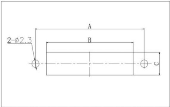
板前安装开孔尺寸
