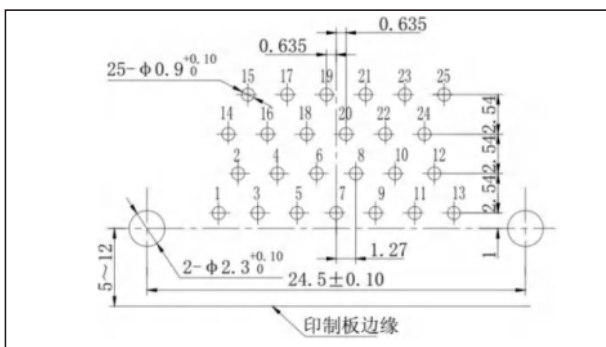
J30J-25ZKW
