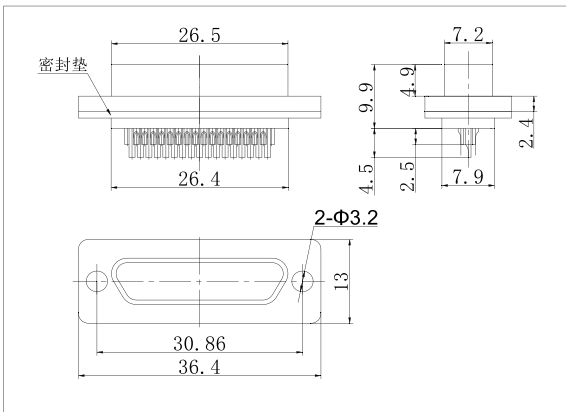
J30JM1-51ZKS
