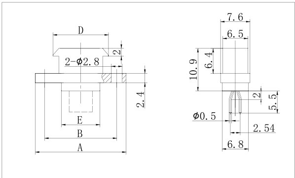
J30JA-9~37ZKN-J
