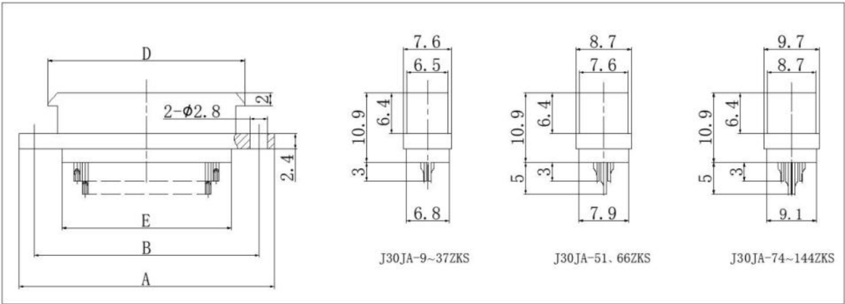
产品外形尺寸图
