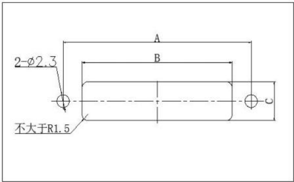
板前安装开孔尺寸
