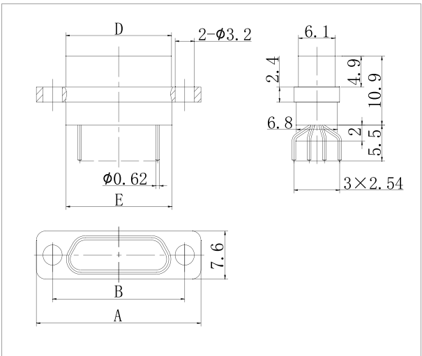
J30J-9~37ZKN
