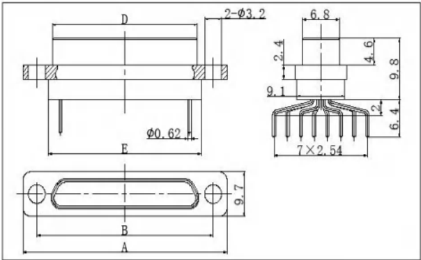
J30J-74~144TJN
