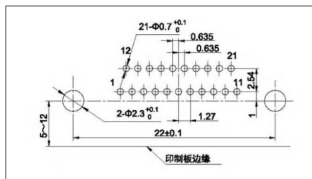
J30J-21ZKW-J
