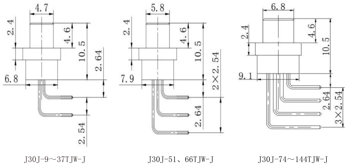
J30J-9~144TJW-J 各芯数插头合件的左视图
