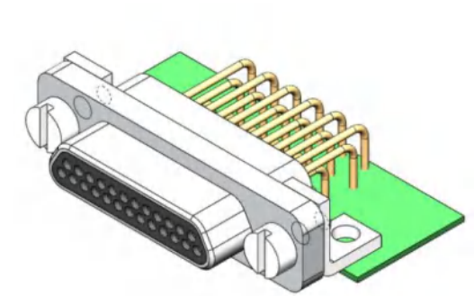
组装示意图
