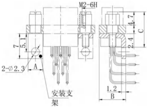
产品外形尺寸图
