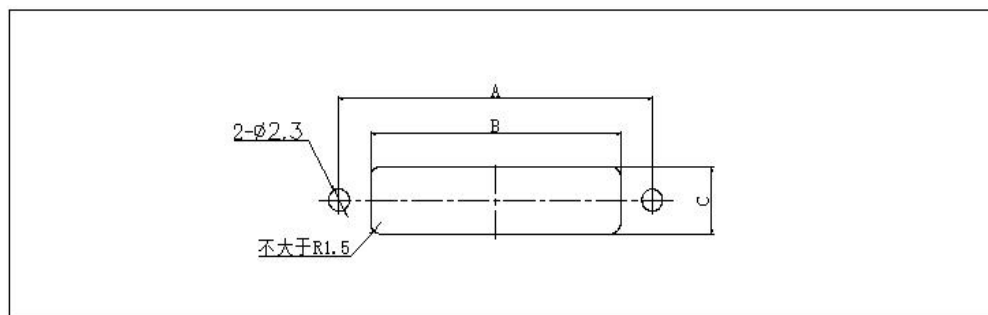
板前安装开孔尺寸
