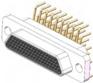
J30J-74TJN
