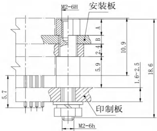
产品外形尺寸图
