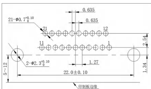
J30JR-21ZJW-J
