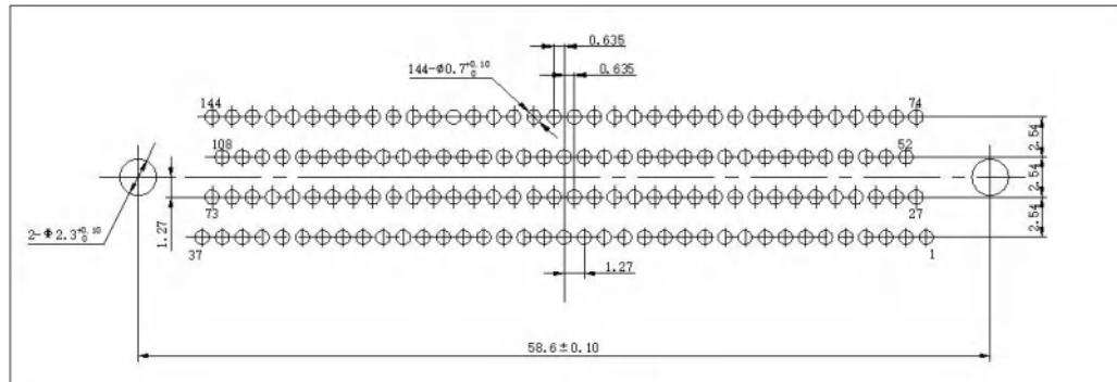
J30J-144TJN□-J
