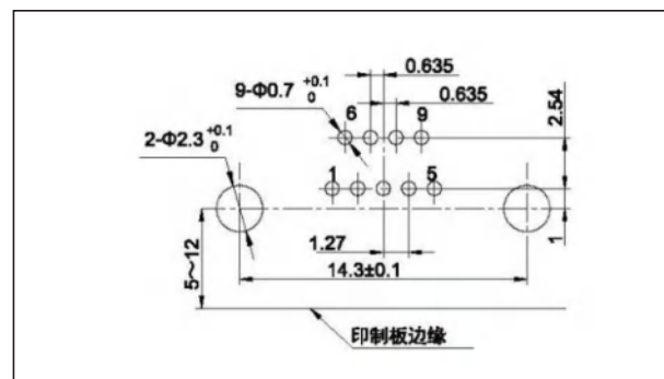
J30J-9ZKW-J
