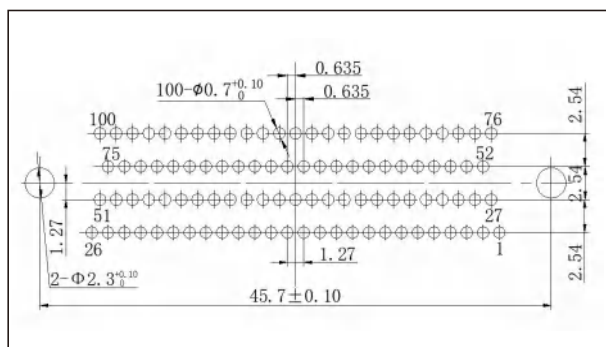
J30J-100TJN□-J
