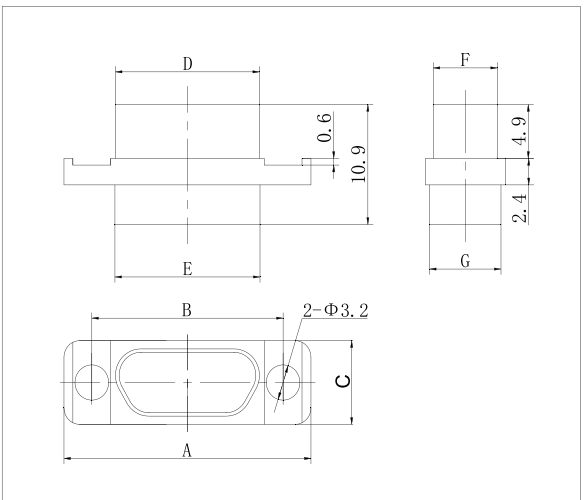
J30J-□ZK-D
