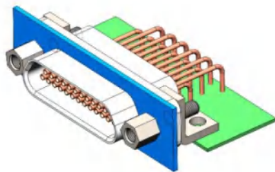
组装示意图
