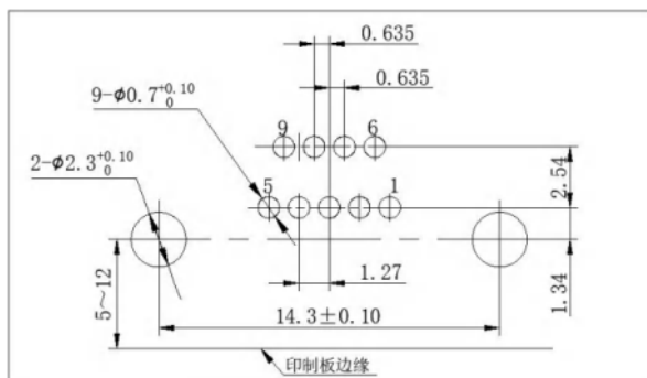
J30JR-9ZJW-J
