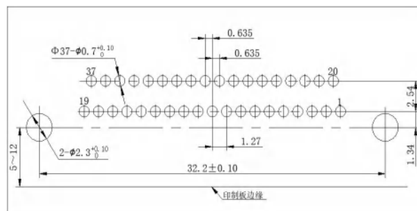
J30JR-37ZJW-J
