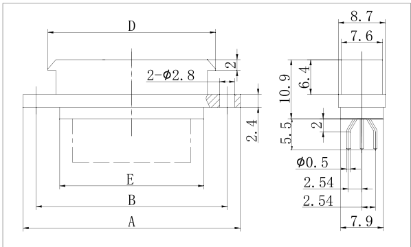
J30JA-51、66ZKN-J
