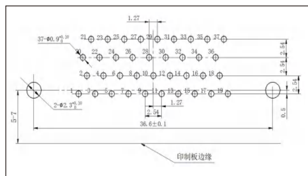
J30JA-37ZKW
