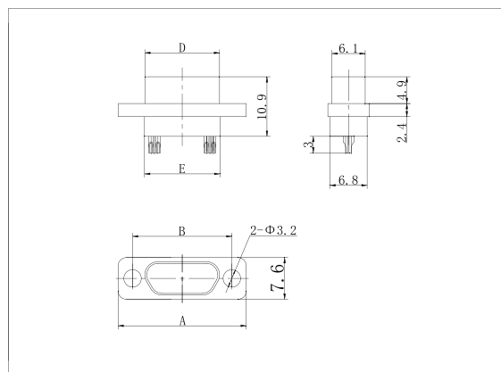
J30J-9~37ZKS
