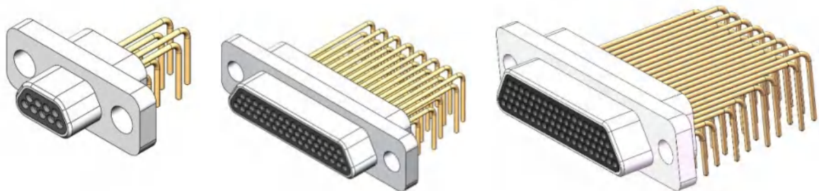
J30J-9TJW
