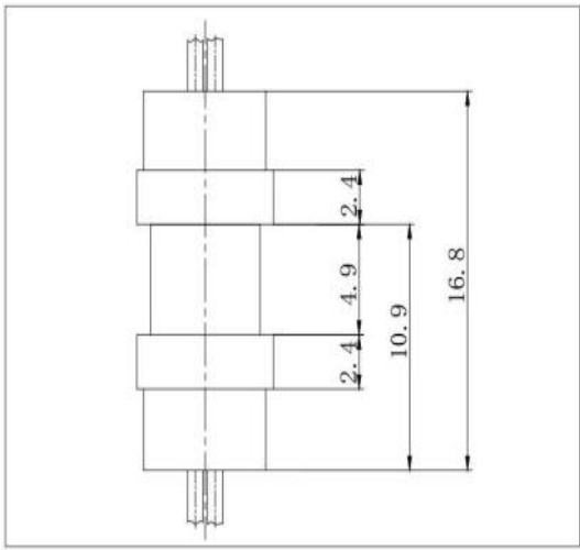
左视图
