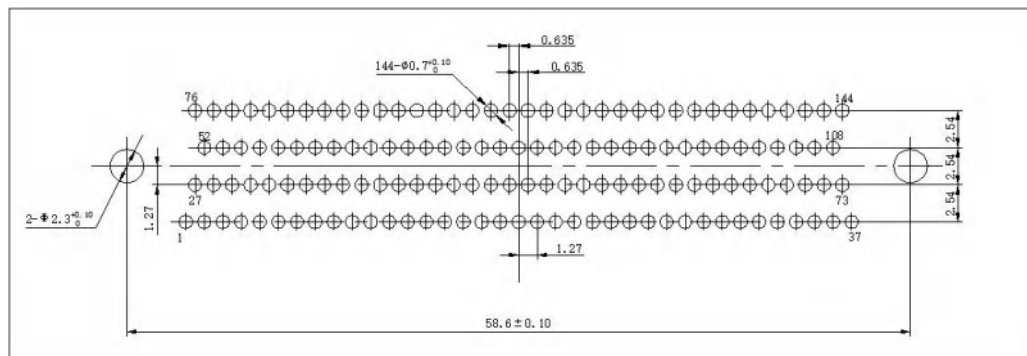
J30J-144ZKN□-J
