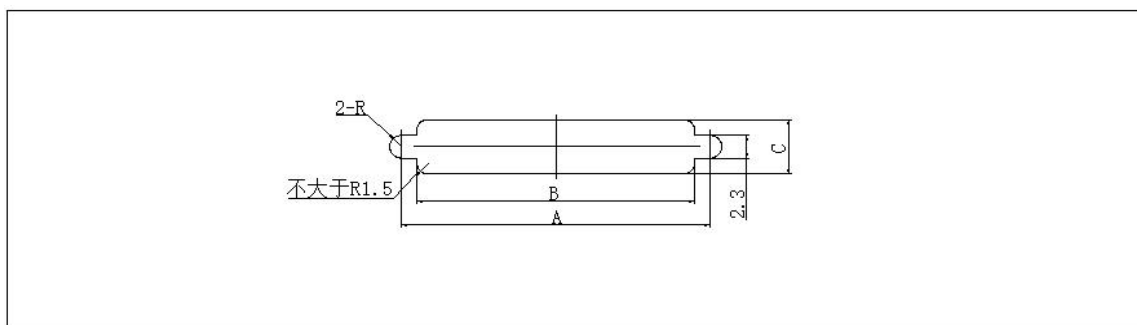
板前安装开孔尺寸
