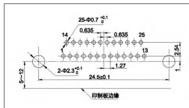
J30J-25ZKW-J
