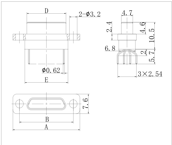
J30J-9~37TJN
