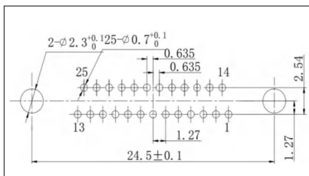
J30J-25TJN□-J
