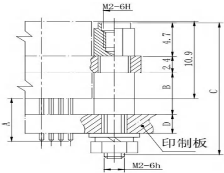
产品外形尺寸图
