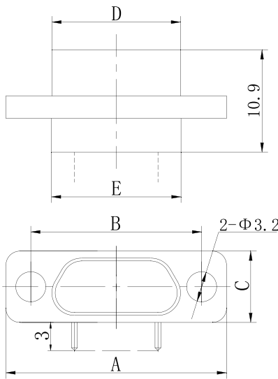
产品外形尺寸图
