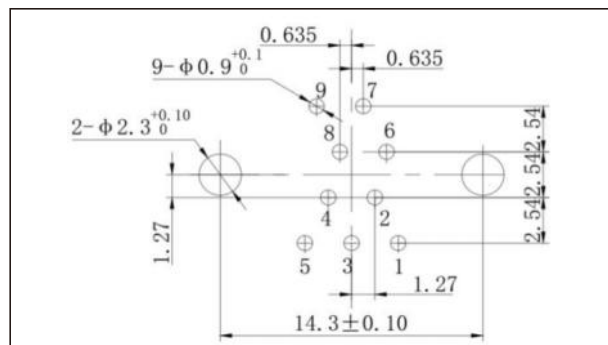
J30J-9TJN□
