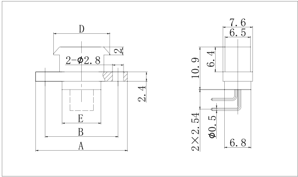
J30JA-9~37ZKW-J
