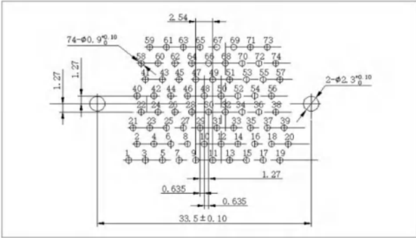
J30JA-74ZKN
