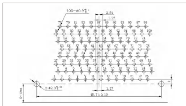
J30J-100ZKW
