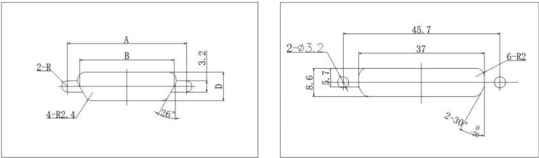
板后安装开孔尺寸（100 芯除外）
