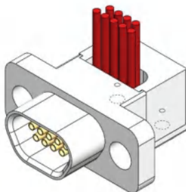
J30J-9ZK-C
