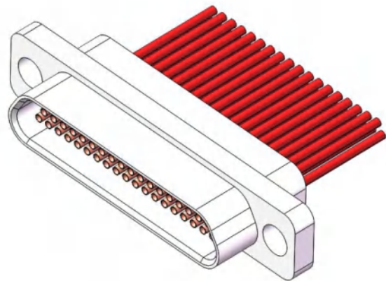
J30J-37ZK(9.6/11.6) 产品外形尺寸图
