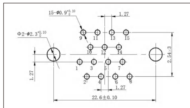
J30JA-15ZKN
