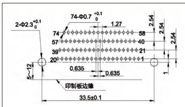
J30J-74TJW-J
