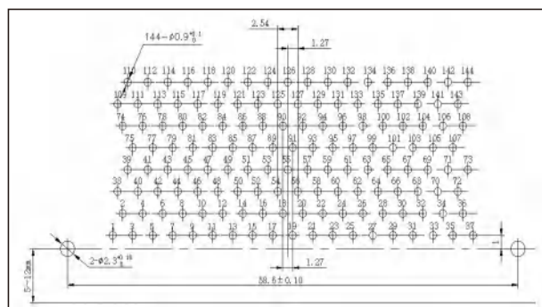
J30J-144ZKW
