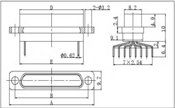
J30J-74~144ZKN
