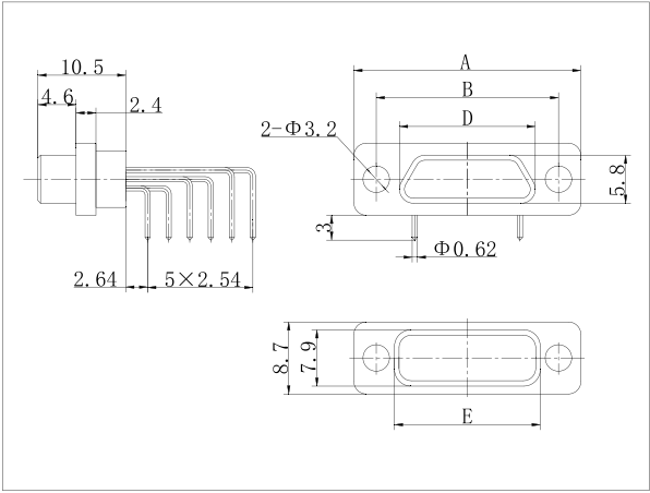
J30J-51、66TJW
