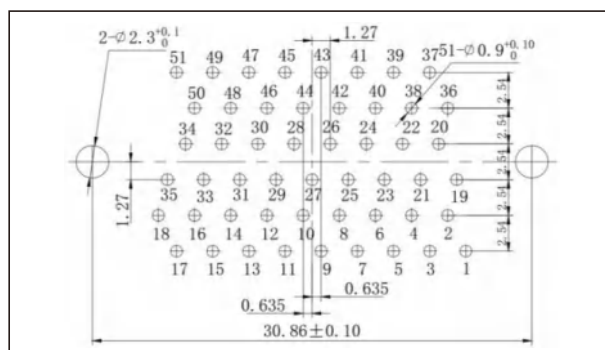
J30J-51TJN□
