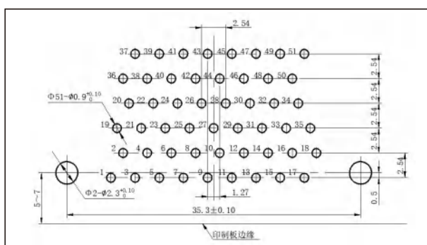
J30JA-51ZKW
