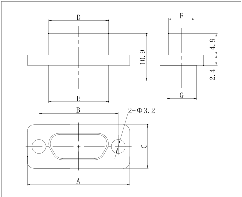
J30J-□ZK-Q8
