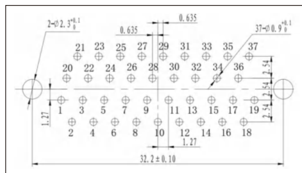
J30J-37ZKN□
