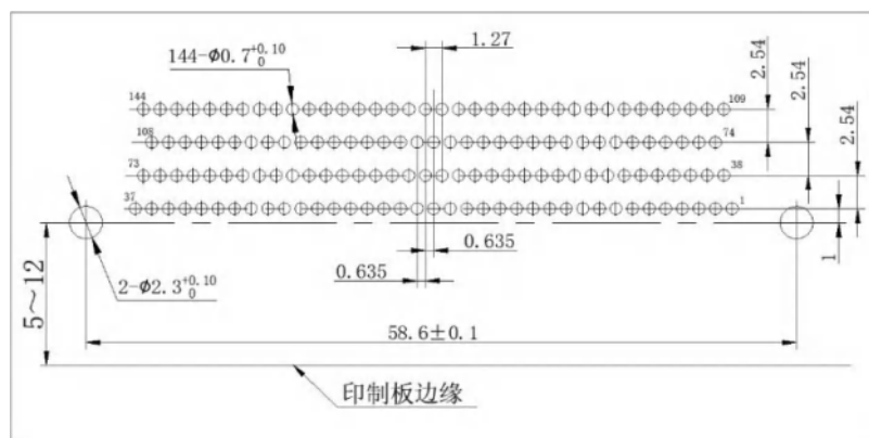
J30J-144TJW-J
