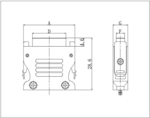
J30JA-□TJ
