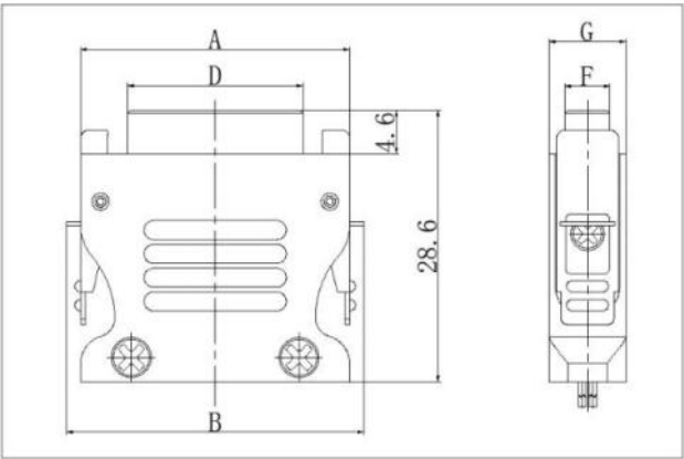
J30JA1-□TJ
