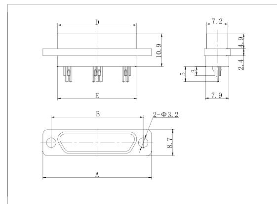
J30J-51~66ZKS
