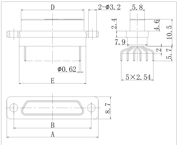
J30J-51、66TJN
