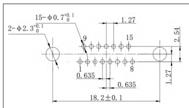
J30J-15ZKN□-J
