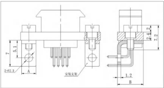
产品外形尺寸图
