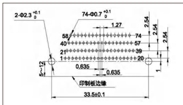
J30J-74ZKW-J
