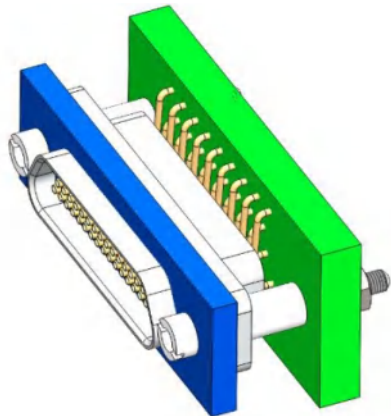
组装示意图
