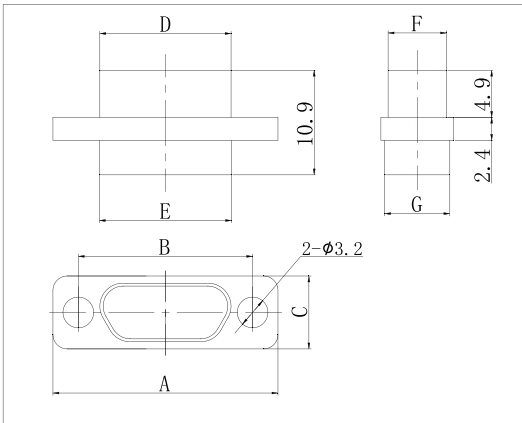
J30J-□ZK(9.6/11.6)
