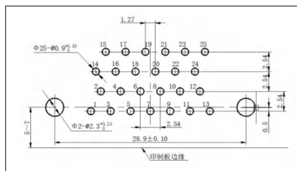
J30JA-25ZKW
