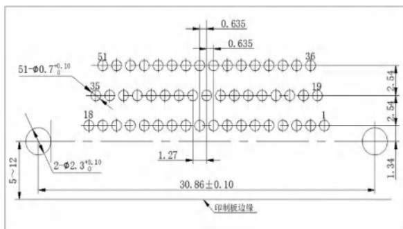
J30JR-51ZJW-J
