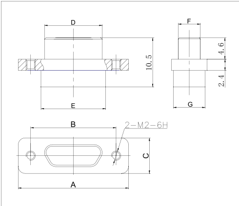
J30JD-□TJ
