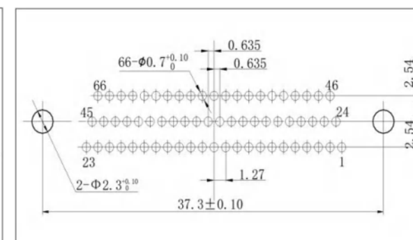
J30JR-66ZJN-J
