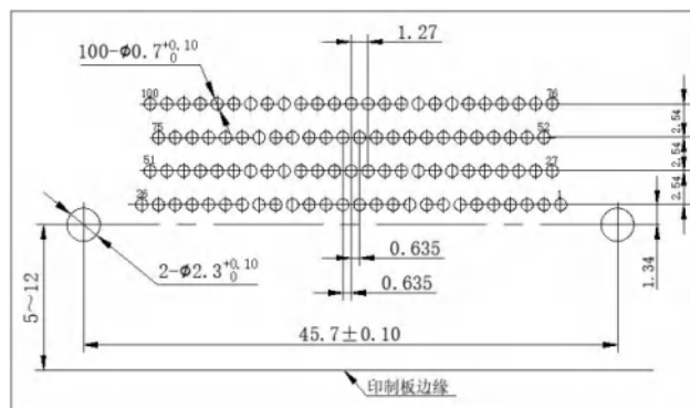
J30JR-100ZJW-J
