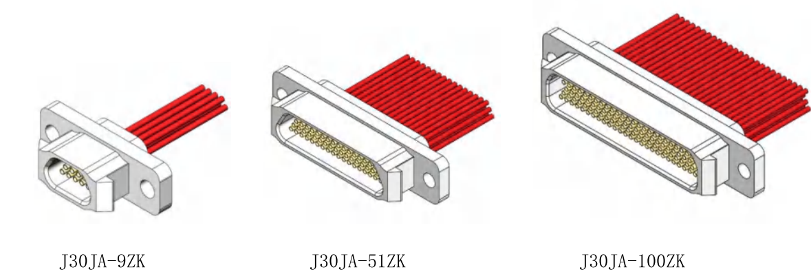
产品外形尺寸图
