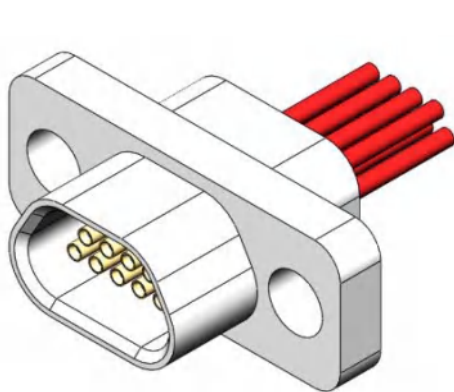
J30J-9ZK(9.6/11.6) 产品外形尺寸图
