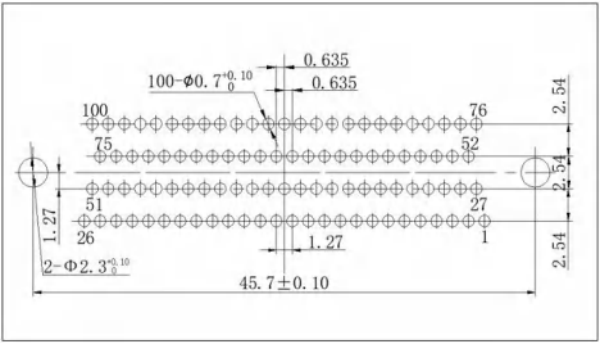
J30JR-100ZJN-J
