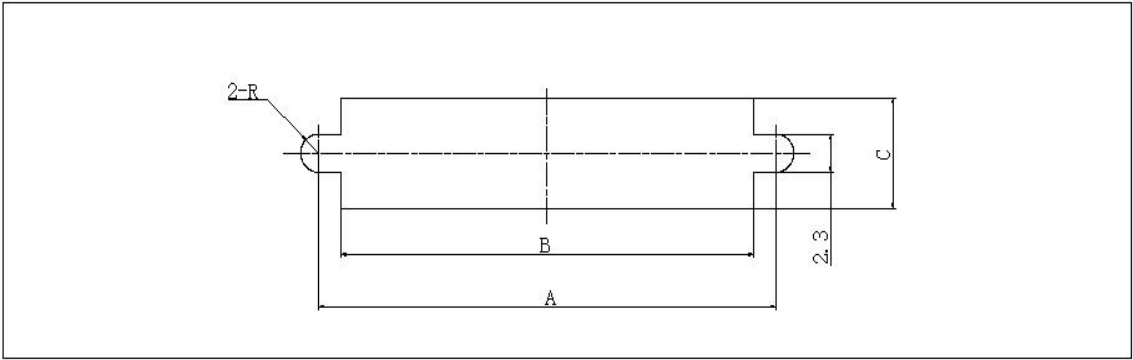
板前安装开孔尺寸
