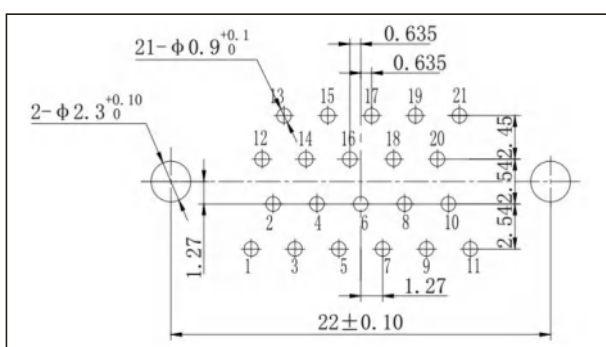
J30J-21ZKN□
