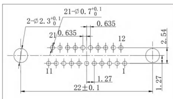
J30JR-21ZJN-J
