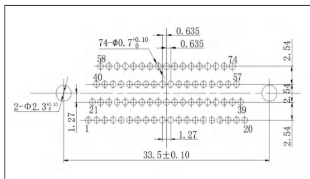
J30J-74ZKN□-J
