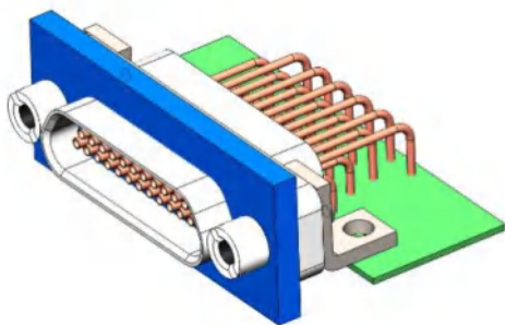
组装示意图
