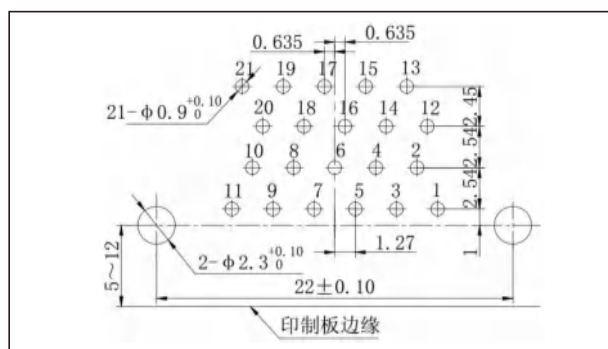
J30J-21TJW
