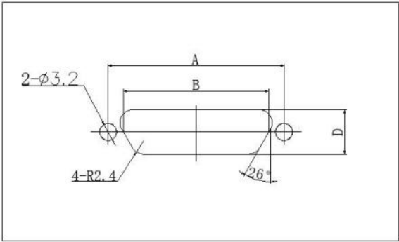
板后安装开孔尺寸（100 除外）
