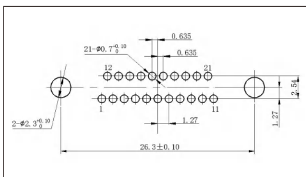
J30JA-21ZKN-J
