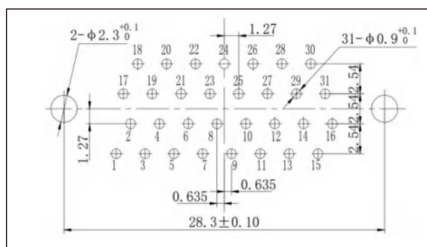
J30J-31ZKN□
