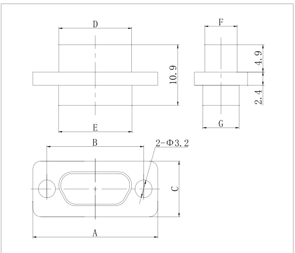
J30J-□ZK-Q
