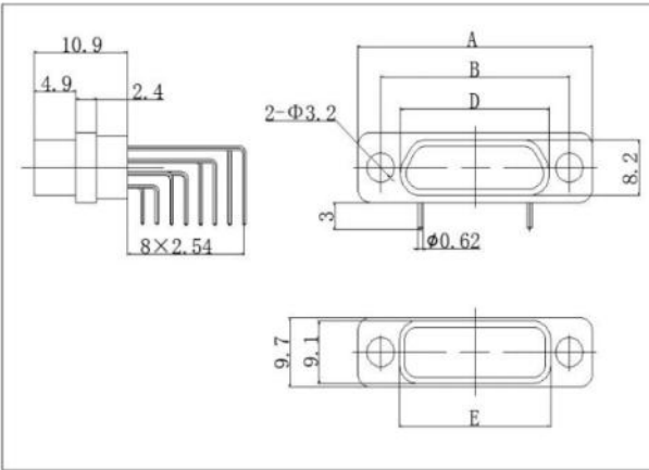
J30J-74~144ZKW
