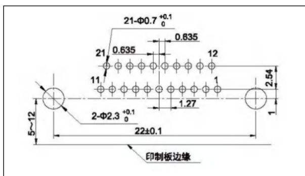
J30J-21TJW-J
