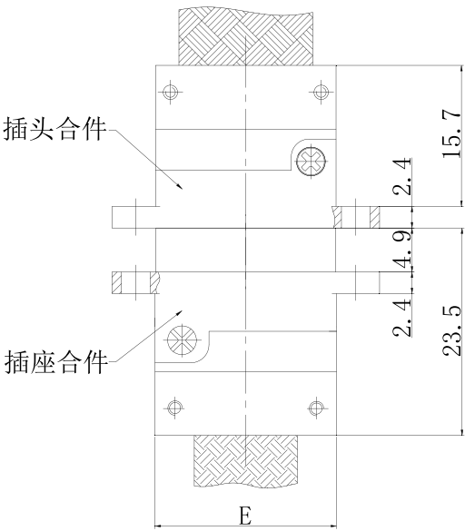
J30J-9~66 芯
