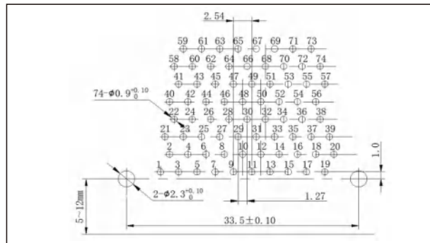
J30J-74ZKW
