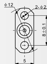
法兰盘尺寸
