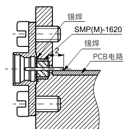
安装示意图
