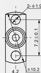
法兰盘尺寸
