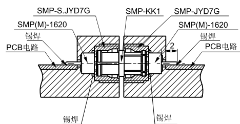
安装示意图
