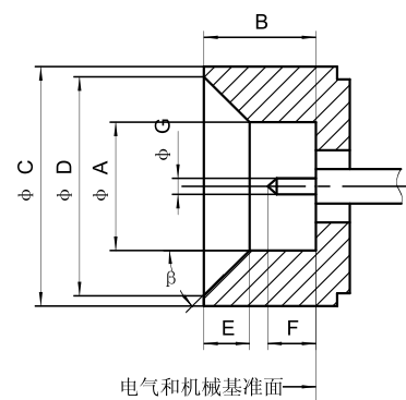
SMP 系列插针接触件连接器界面 (光孔带制动装置)
