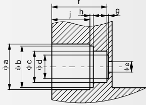
建议安装开孔尺寸
