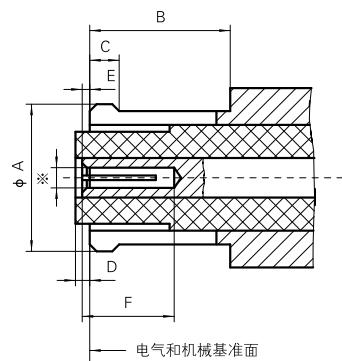
※ 可插入直径为 φ 0.38 ± 0.03 的插针。 SMP 系列插孔接触件连接器界面
