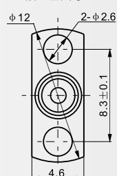
法兰盘尺寸
