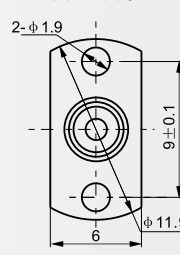
法兰盘尺寸
