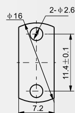
法兰盘尺寸
