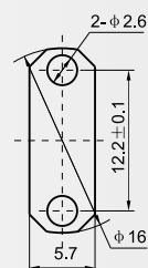
法兰盘尺寸
