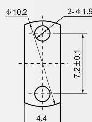
法兰盘尺寸
