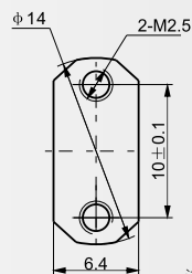
法兰盘尺寸
