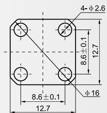
法兰盘尺寸
