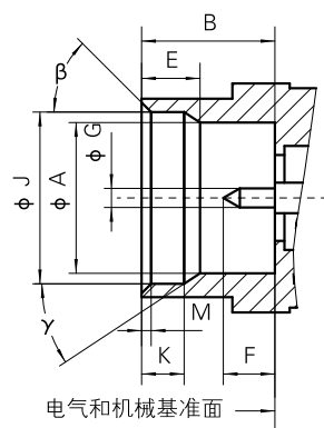
SMP 系列插针接触件连接器界面 (光孔)
