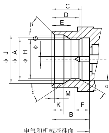
SMP 系列插针接触件连接器界面 (全擒纵或有限擒纵)
