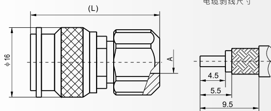
电缆剥线尺寸
