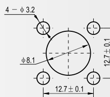
建议安装开孔尺寸
