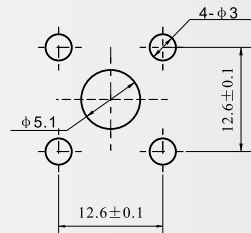
建议安装开孔尺寸
