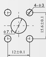
建议安装开孔尺寸
