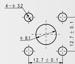
建议安装开孔尺寸
