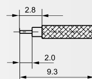
电缆剥线尺寸
