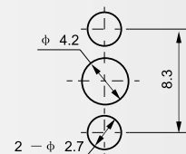
建议安装开孔尺寸
