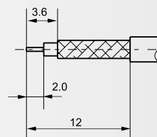
电缆剥线尺寸
