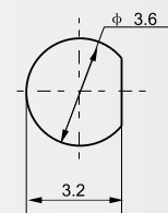
建议安装开孔尺寸
