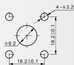
建议安装开孔尺寸
