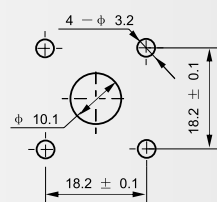
建议安装开孔尺寸
