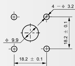
建议安装开孔尺寸
