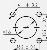
建议安装开孔尺寸
