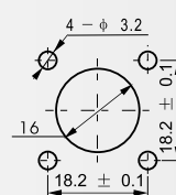
建议安装开孔尺寸
