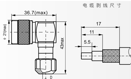
电缆剥线尺寸
