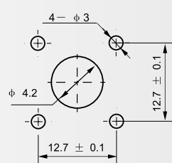
建议安装开孔尺寸
