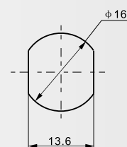
建议安装开孔尺寸
