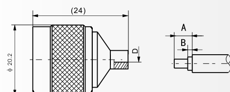
电缆剥线尺寸
