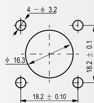
建议安装开孔尺寸
