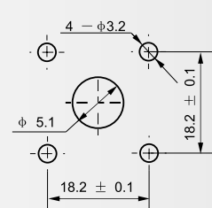
建议安装开孔尺寸
