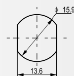
建议安装开孔尺寸
