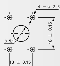
建议安装开孔尺寸
