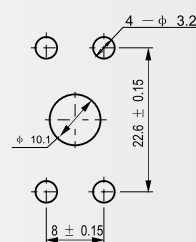
建议安装开孔尺寸
