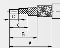
电缆剥线尺寸
